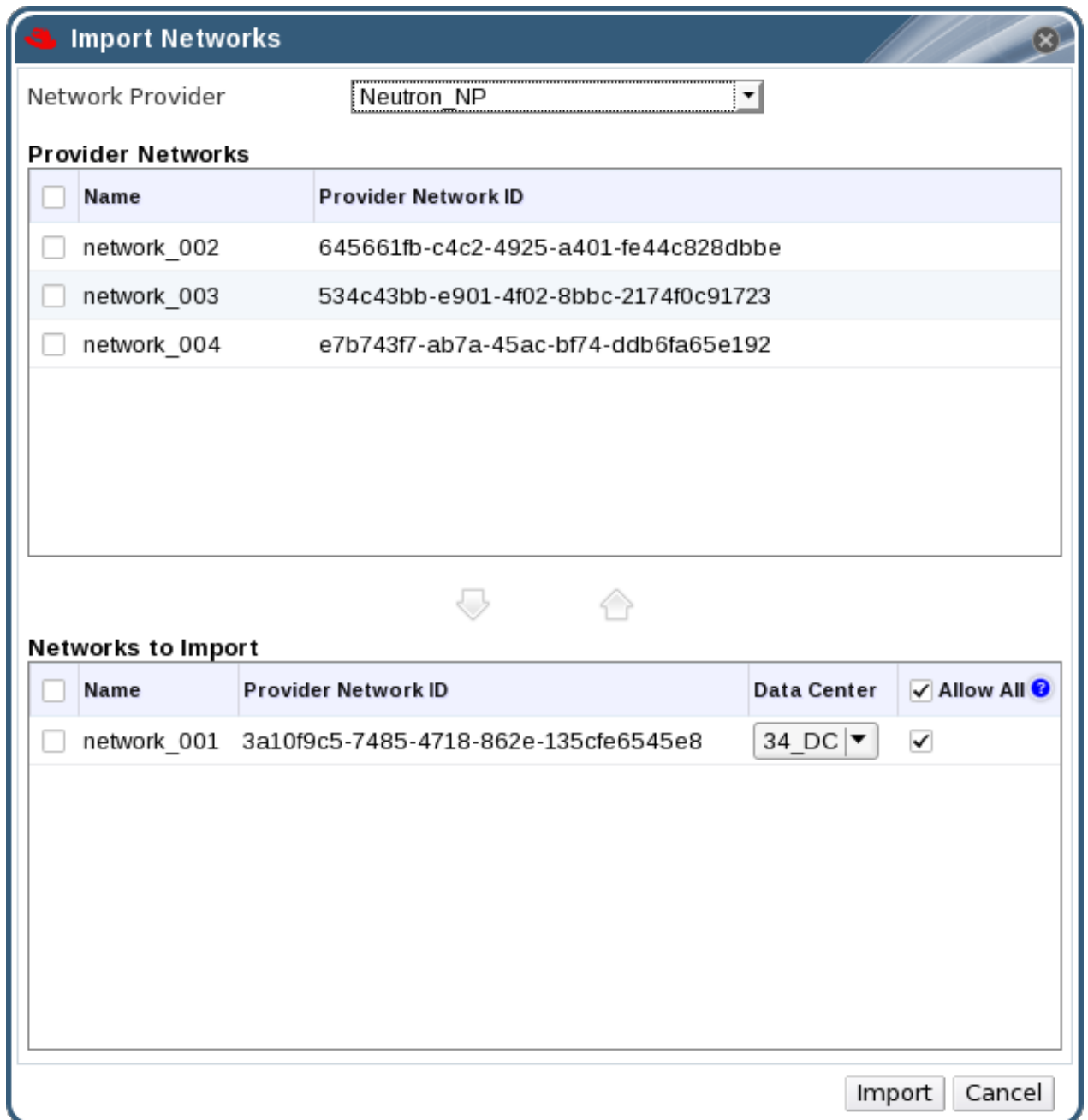
図5.3 ネットワークのインポートウィンドウ
