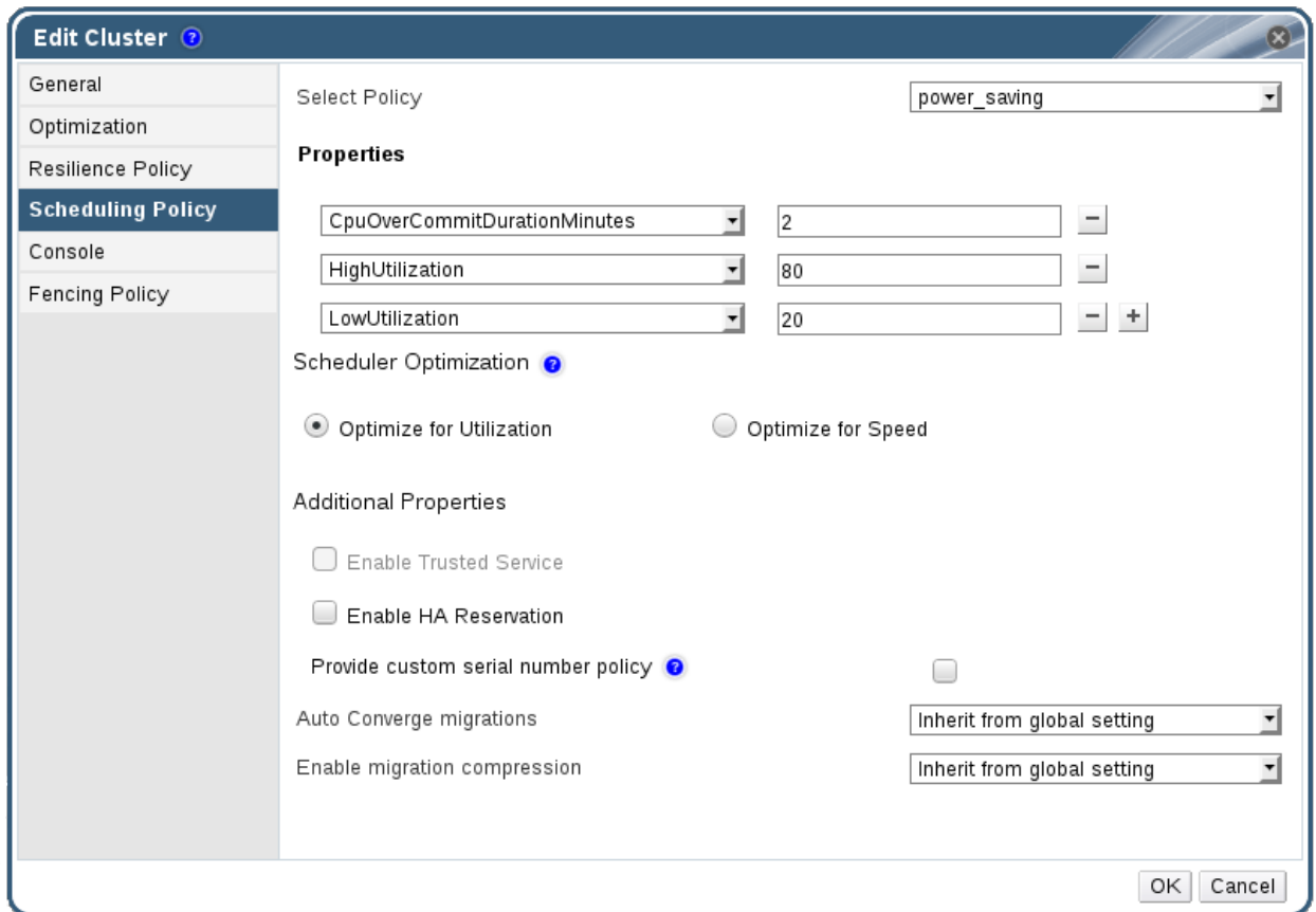
図4.4 スケジューリングポリシーの編集
