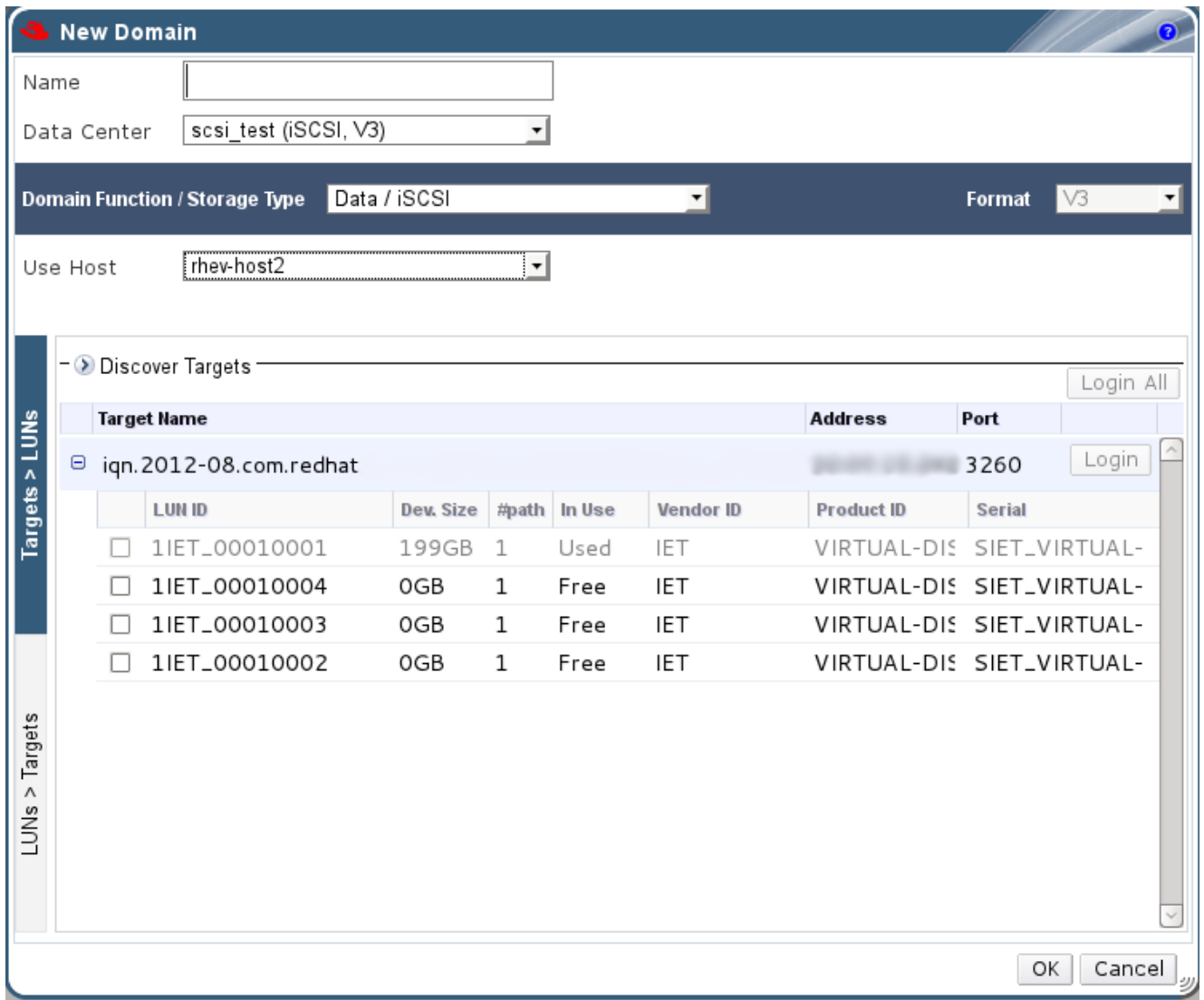
図7.6 Red Hat Virtualization 管理ポータルで使用できない LUN
