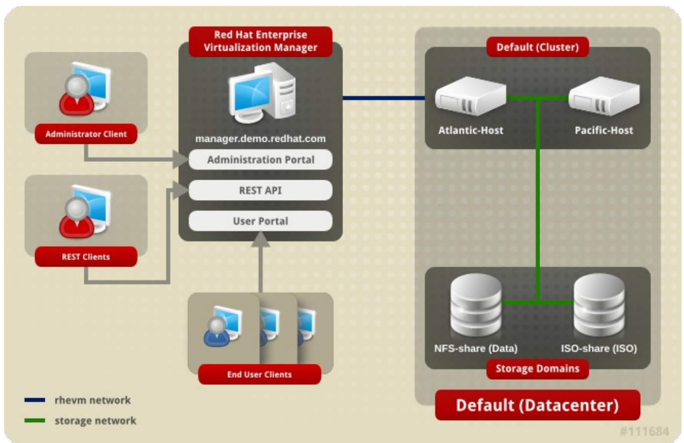
図3.1 データセンター
