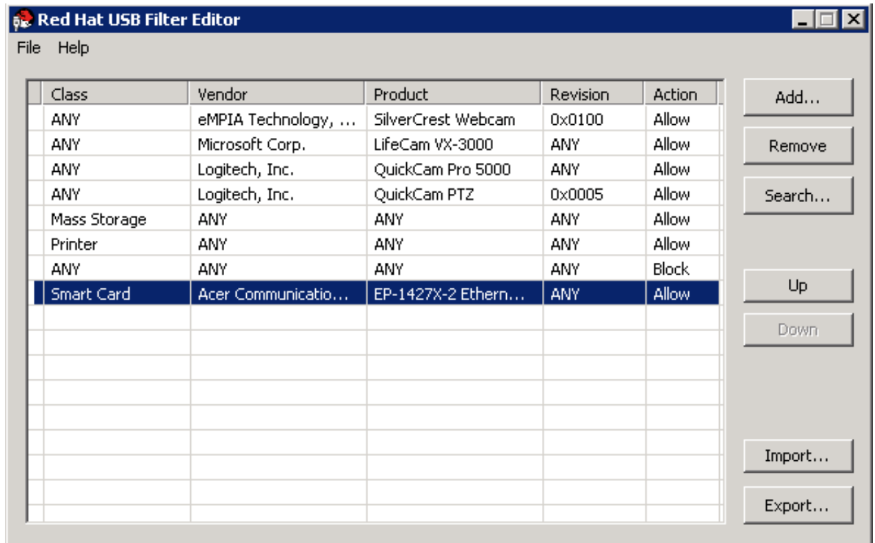
図17.3 USB ポリシーの選択
