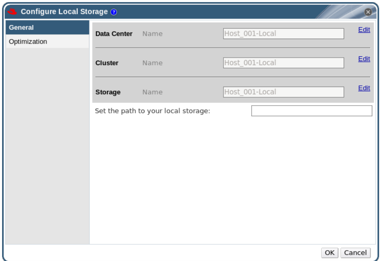
図7.2 ローカルストレージの設定ウィンドウ
