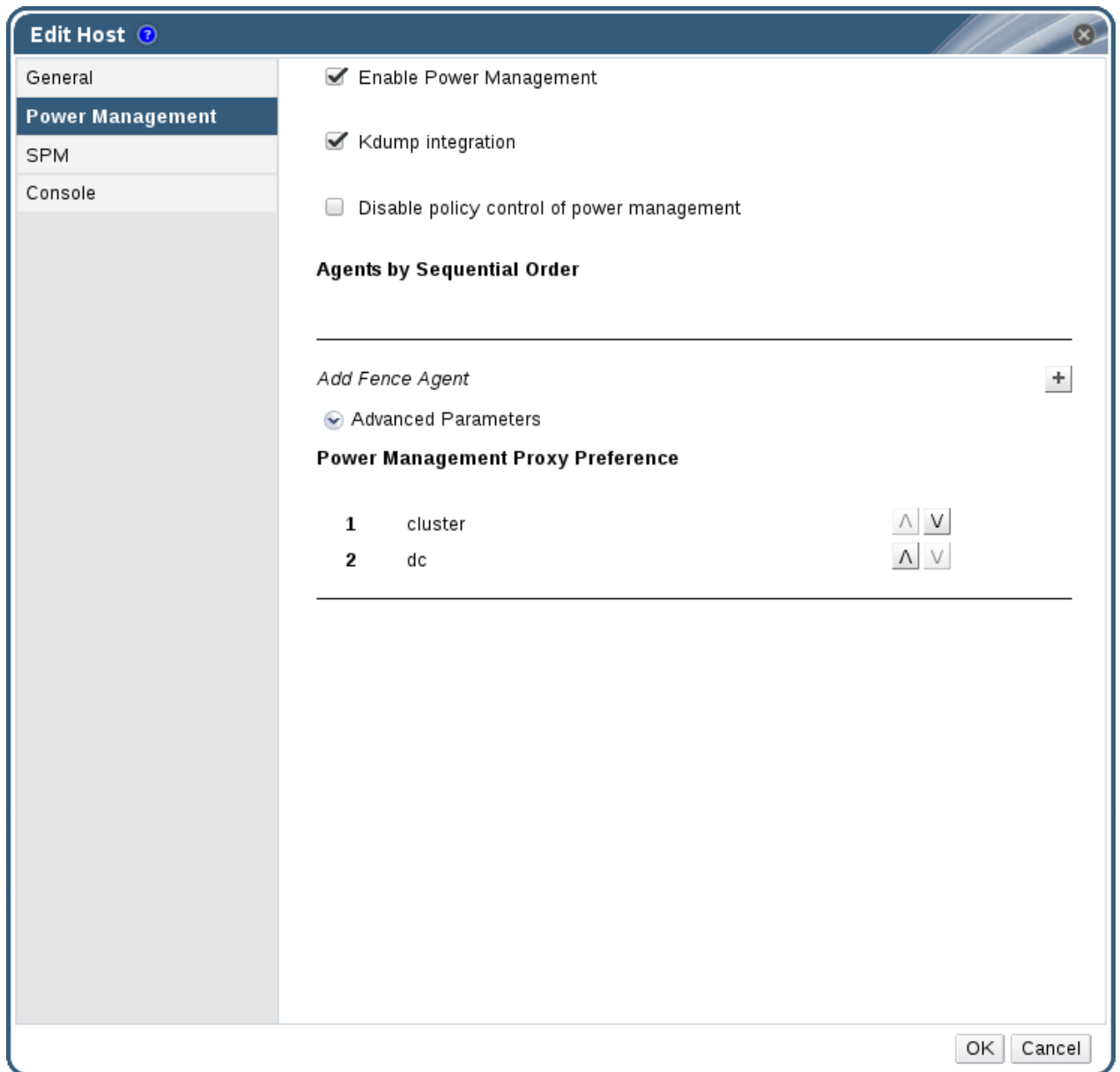
図6.2 電源管理の設定
