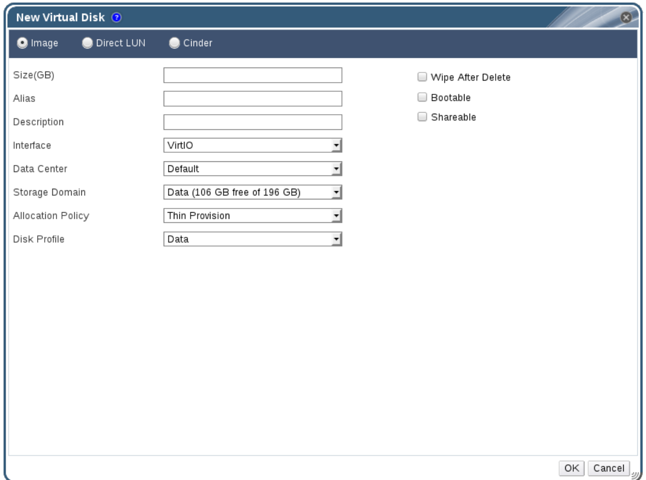
図10.1 仮想ディスクの追加ウィンドウ
