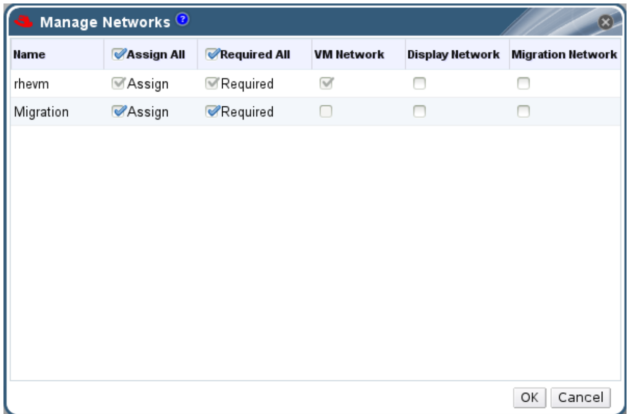
図5.1 ネットワークの管理
