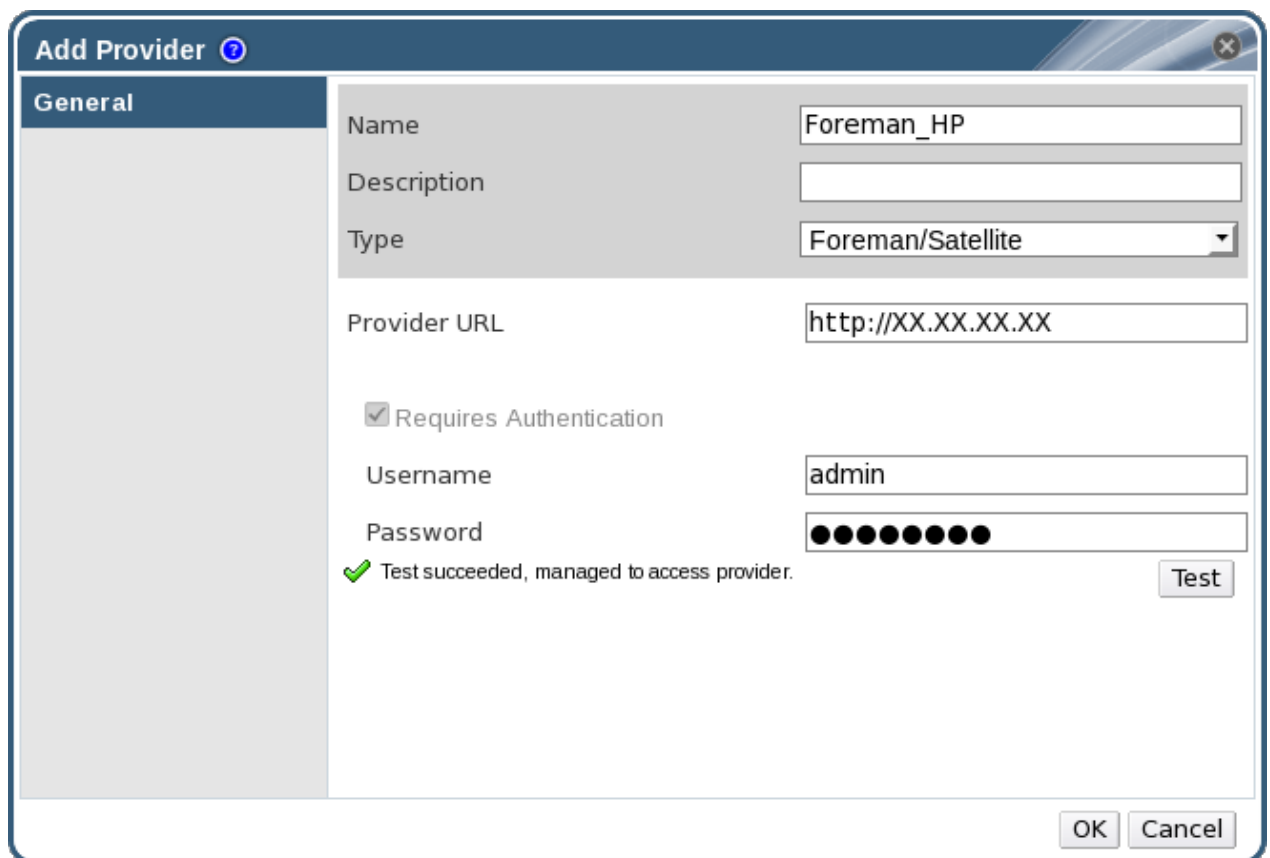
図11.1 プロバイダーの追加ウィンドウ
