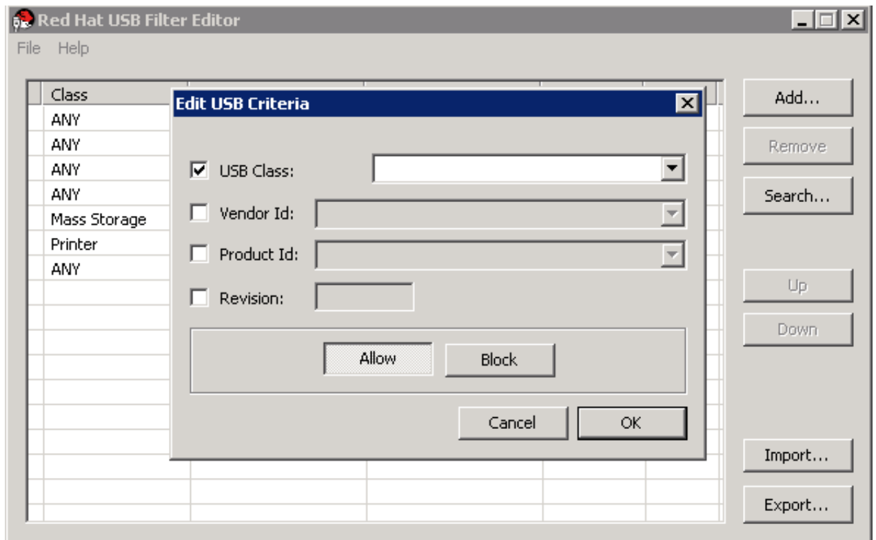
図17.2 USB Criteria の編集
