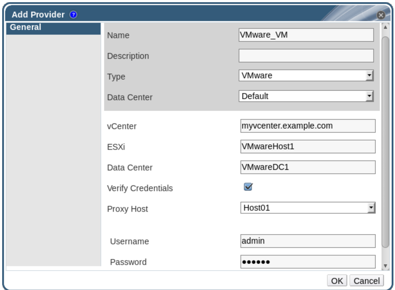
図11.6 プロバイダーの追加ウィンドウ
