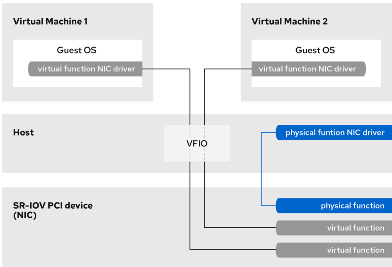
图 11.1. SR-IOV 架构
