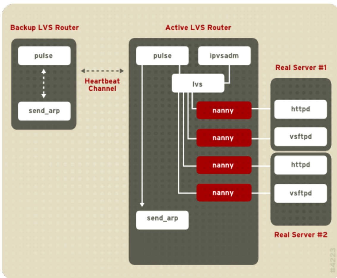
圖形 1.5. LVS Components
