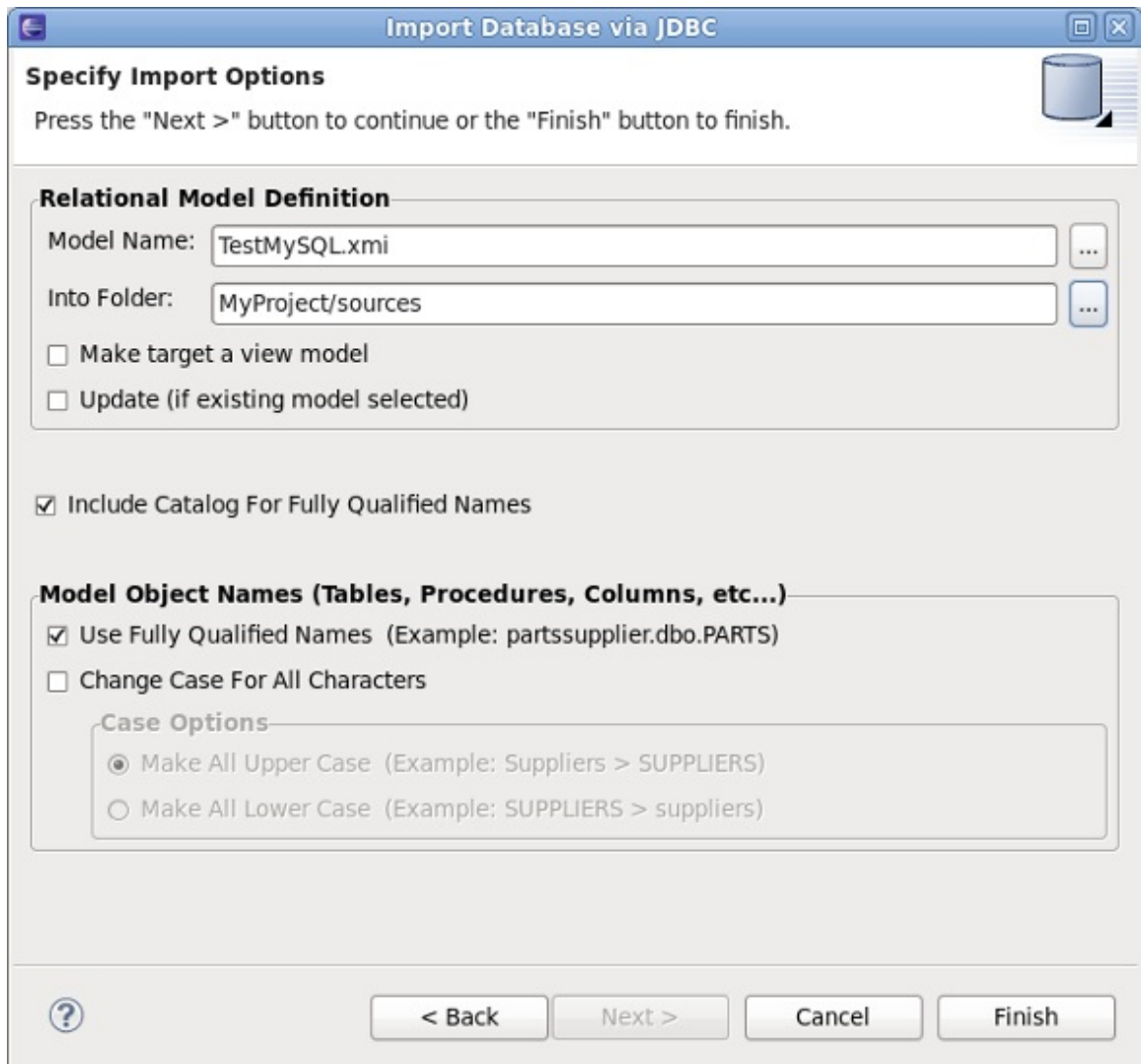
Figure 7.10. Import Options
