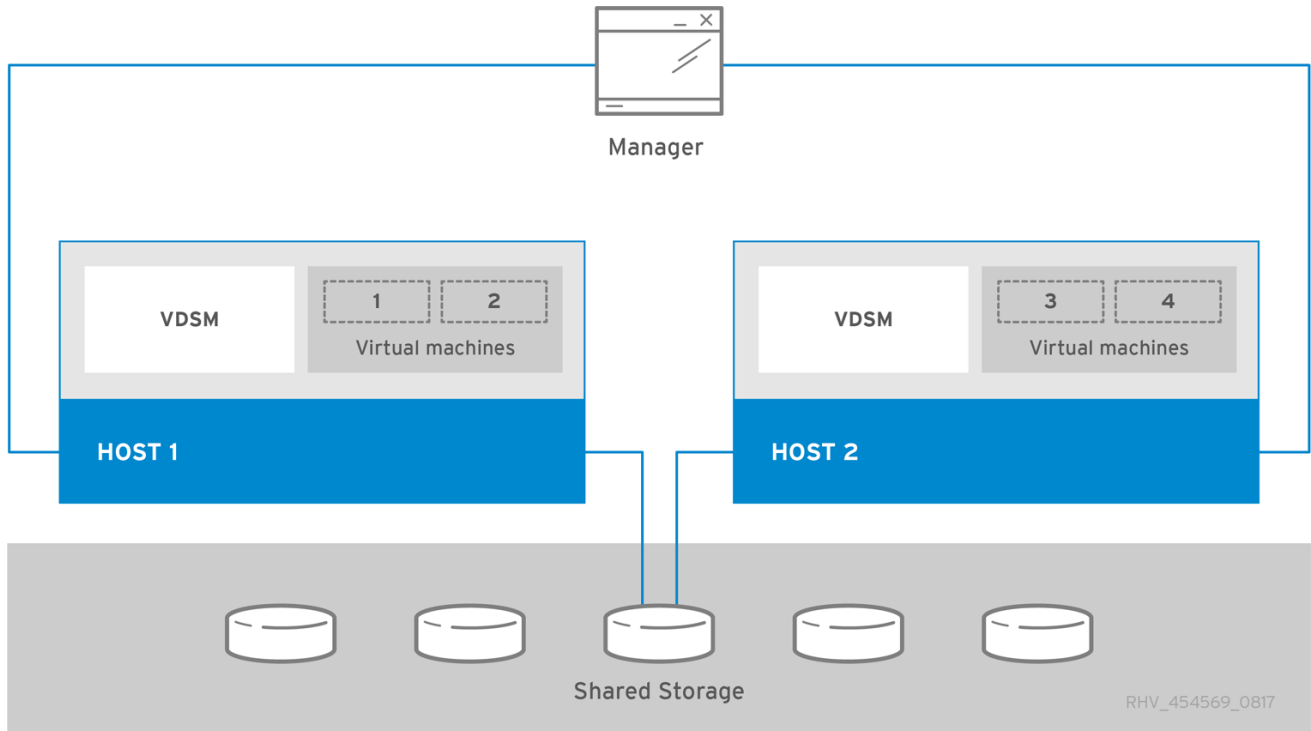
図1 スタンドアロンの Manager の Red Hat Virtualization アーキテクチャー
