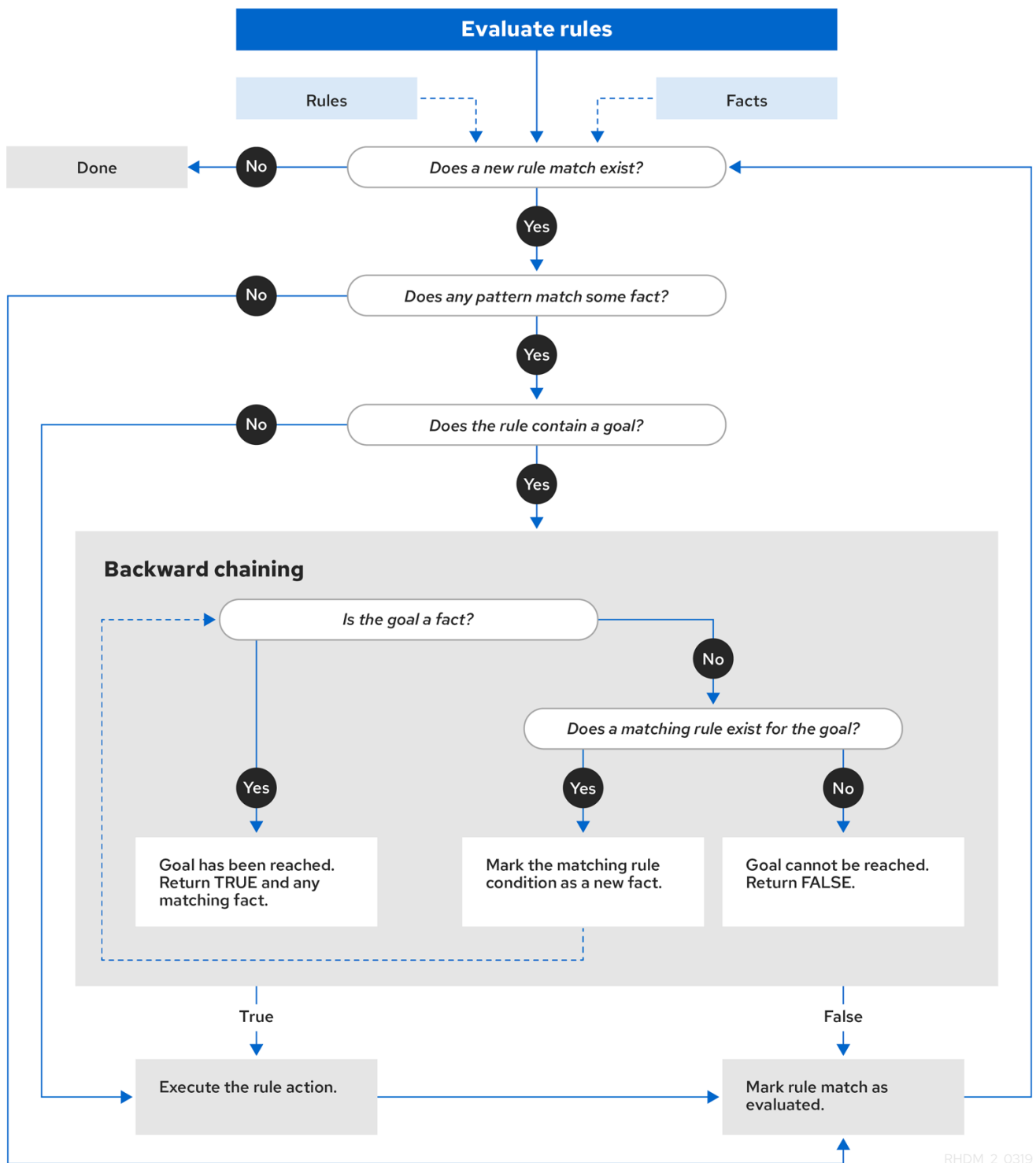
図89.4 前向き連鎖と後向き連鎖を使用したルール評価のロジック
