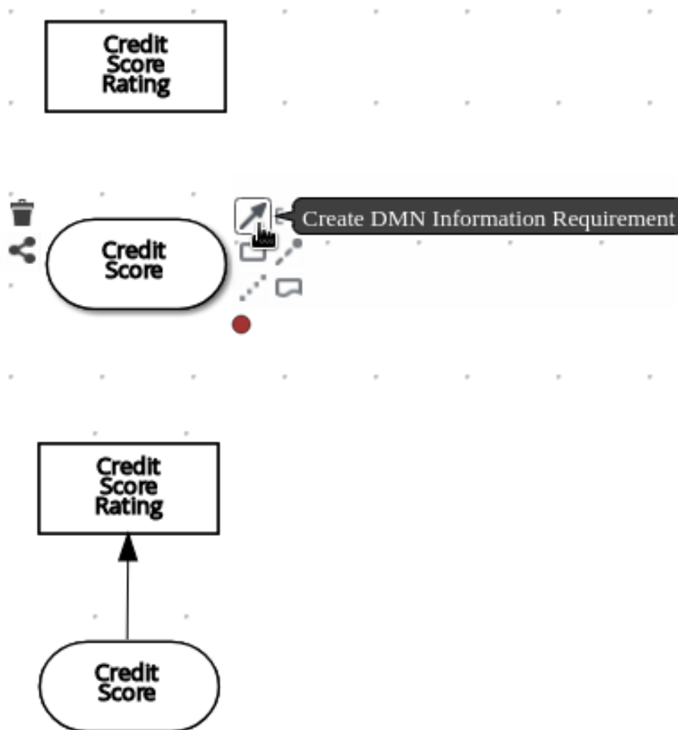
図6.8 クレジットスコアの入力からクレジットスコア評価のデシジョンへの接続
