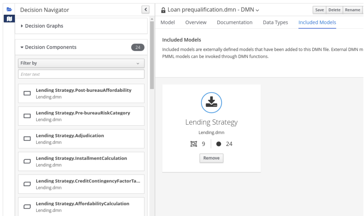
図6.40 追加した DMN モデルのデシジョンコンポーネントを含む DMN ファイル
