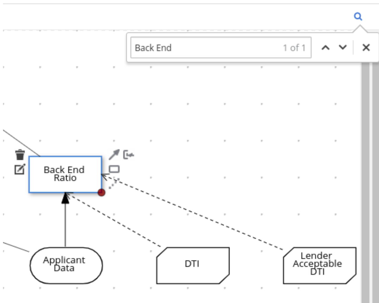
図6.64 DRD 検索
