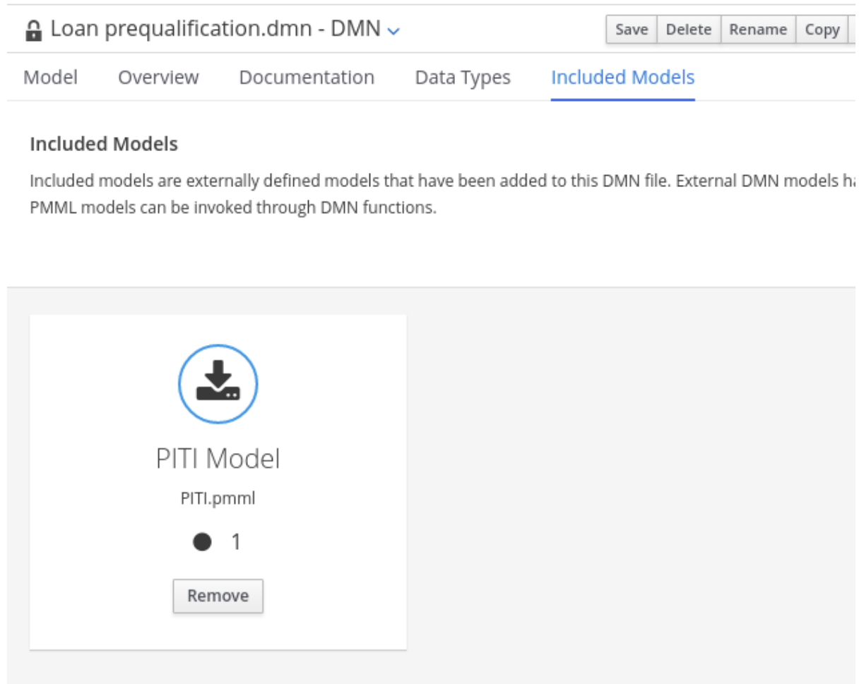
図6.44 PMML モデルを含む DMN ファイル
