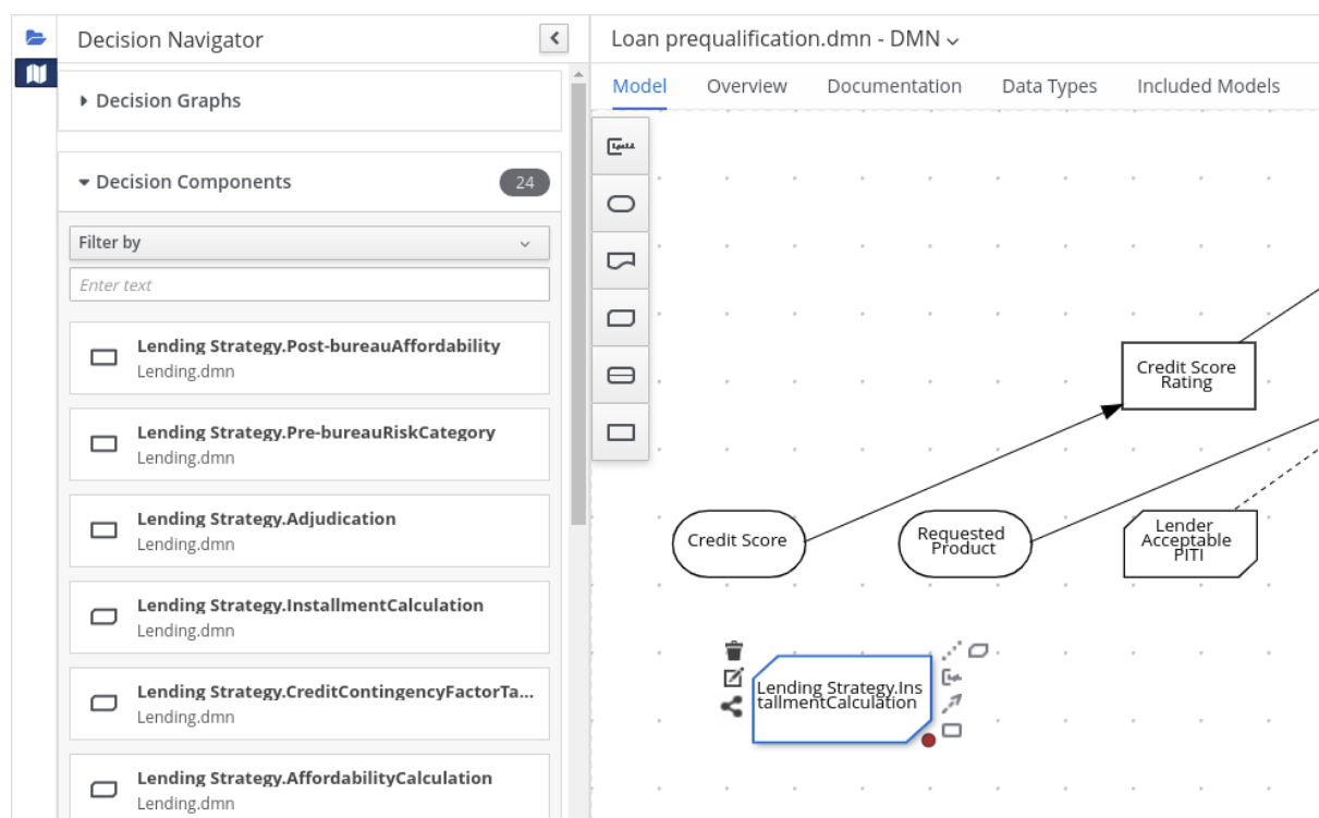
図6.42 追加した DMN モデルの DRD コンポーネントの追加
