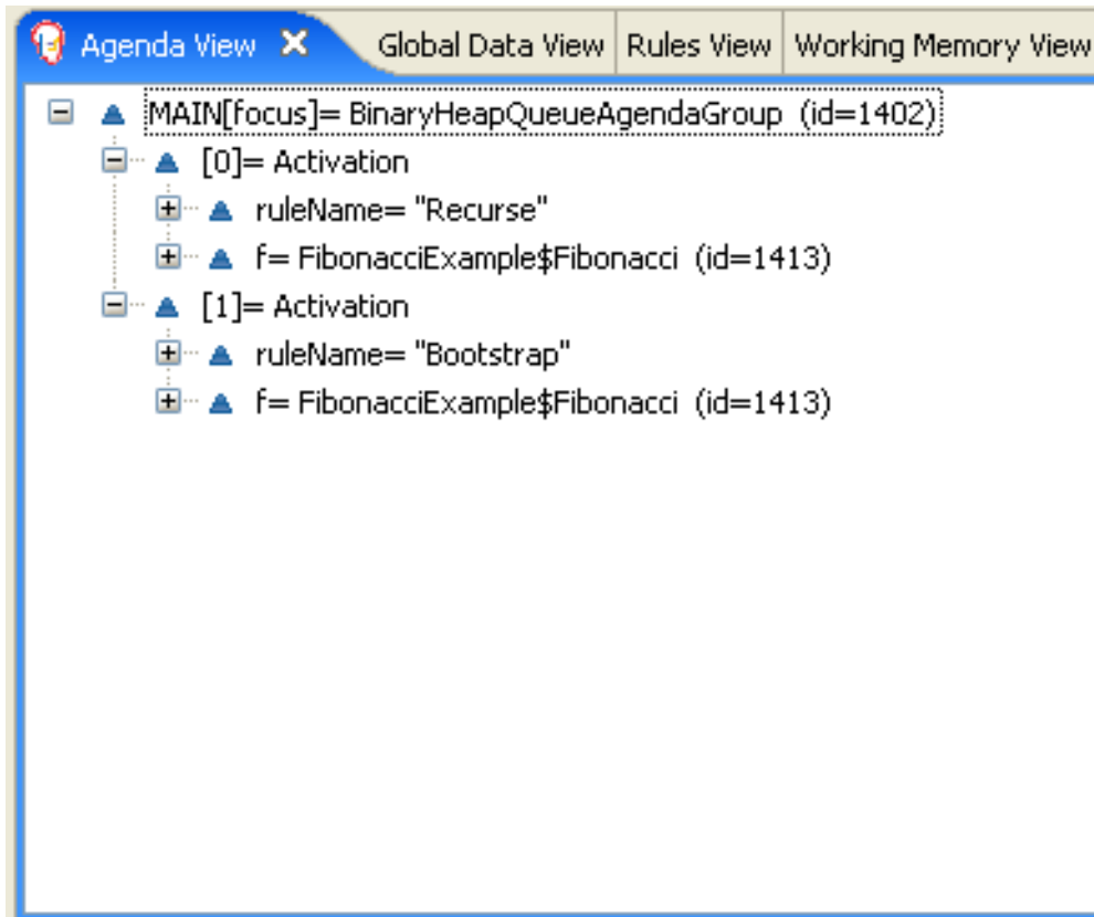
図21.8 アジェンダビュー 1 でのルール "Recurse" および "Bootstrap"
