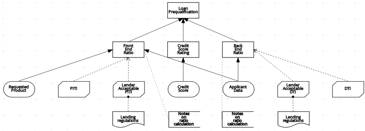
図6.51 ローンの事前審査のための単一の DRD
