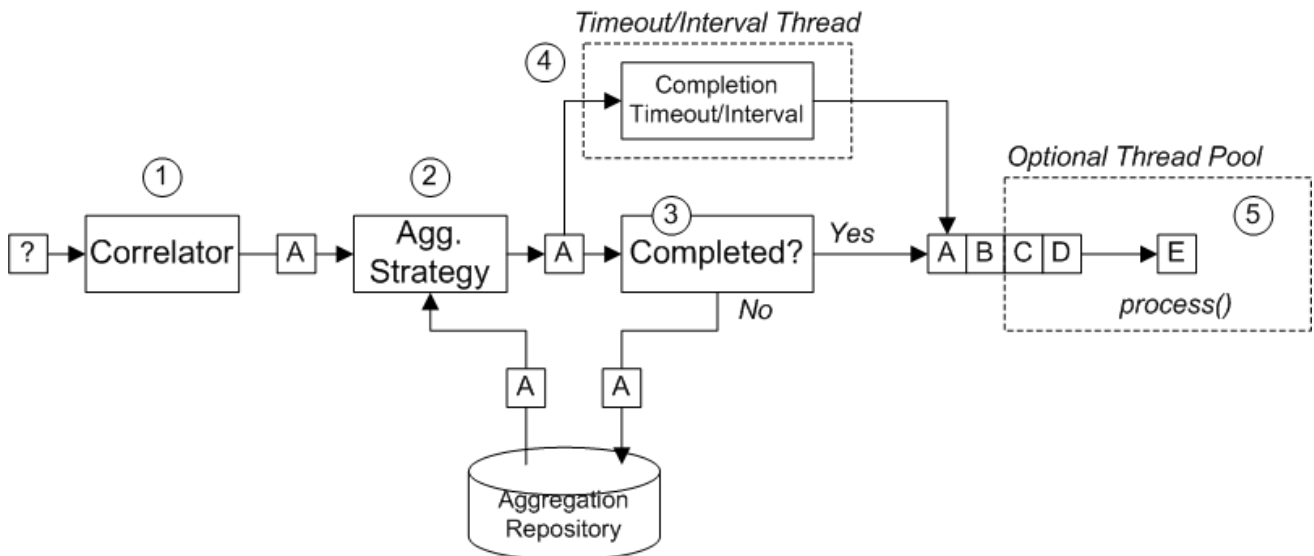
図8.6 Aggregator の実装
