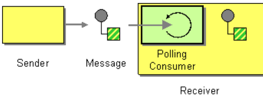
図11.2 Polling Consumer パターン
