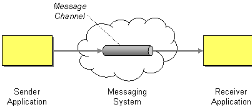
図5.2 Message Channel パターン
