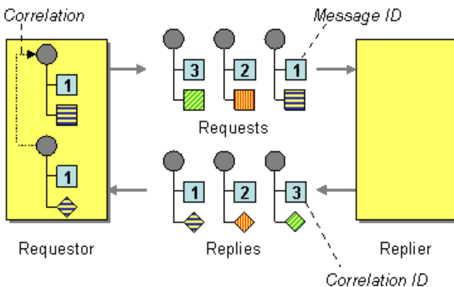
図7.1相関識別子パターン
