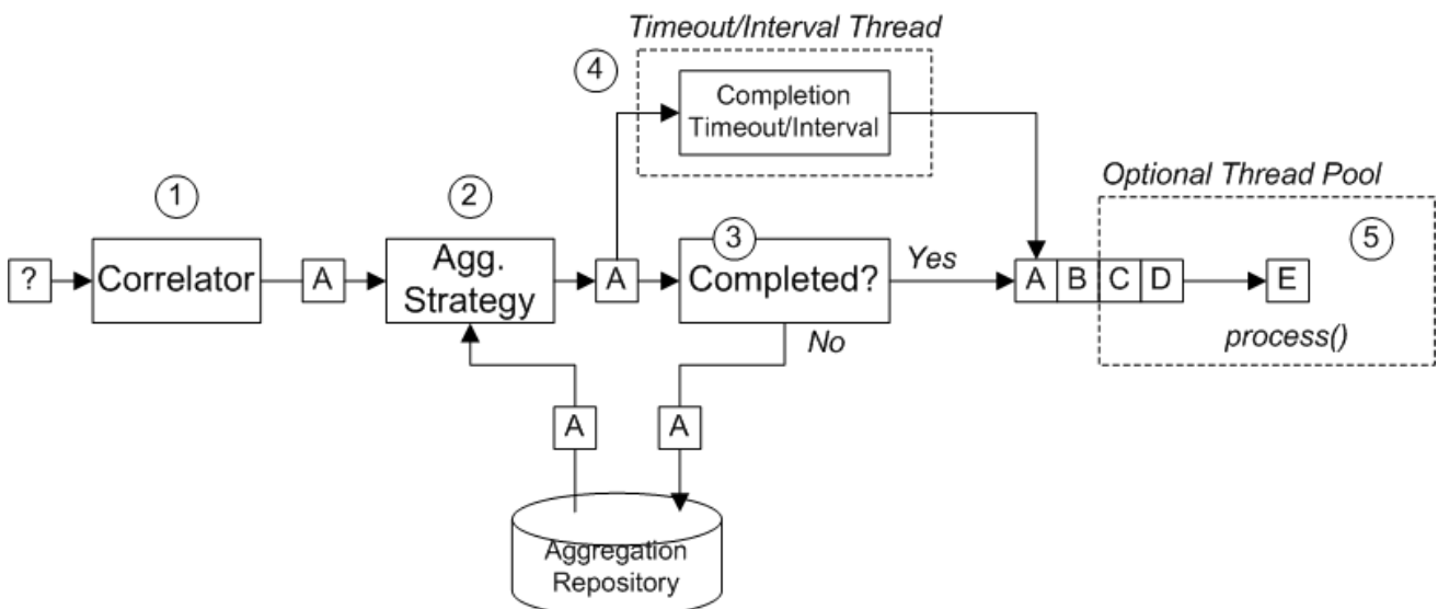
図8.6 Aggregator の実装
