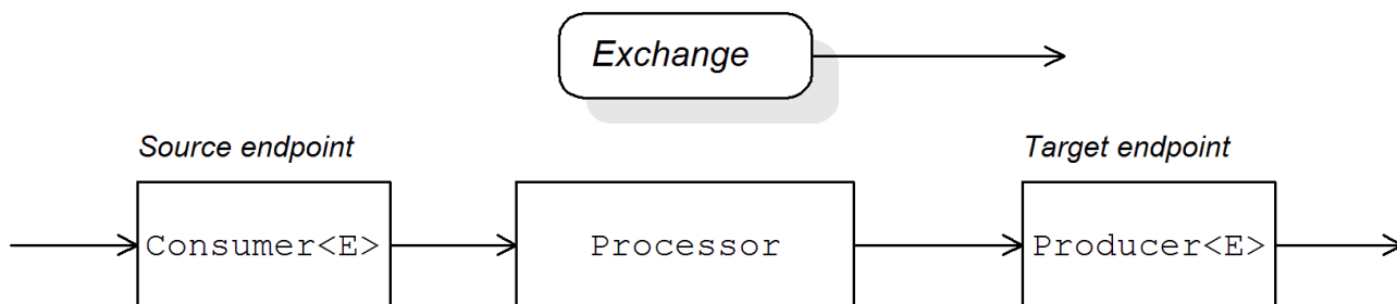
図38.2 ルートのコシューマーおよびプロデューサーインスタンス
