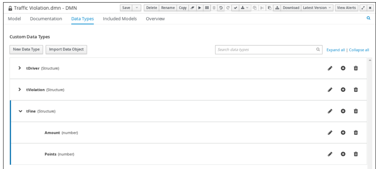
図3.7 tFine のカスタムデータタイプ
