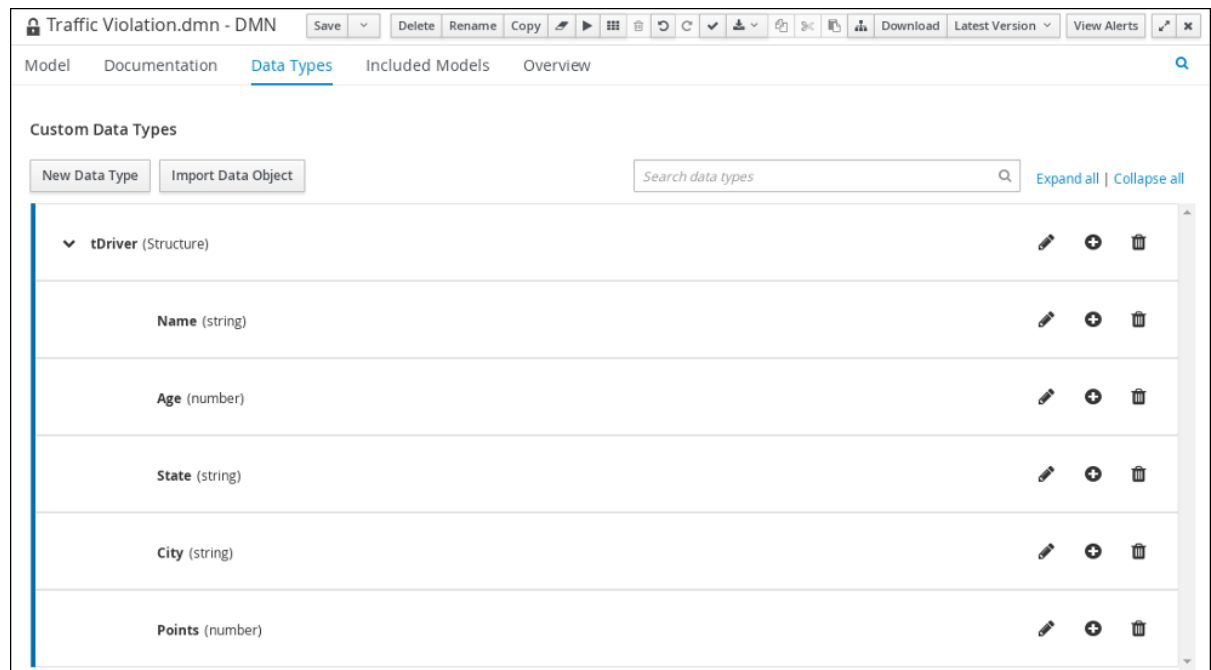
図3.5 tDriver のカスタムデータタイプ
