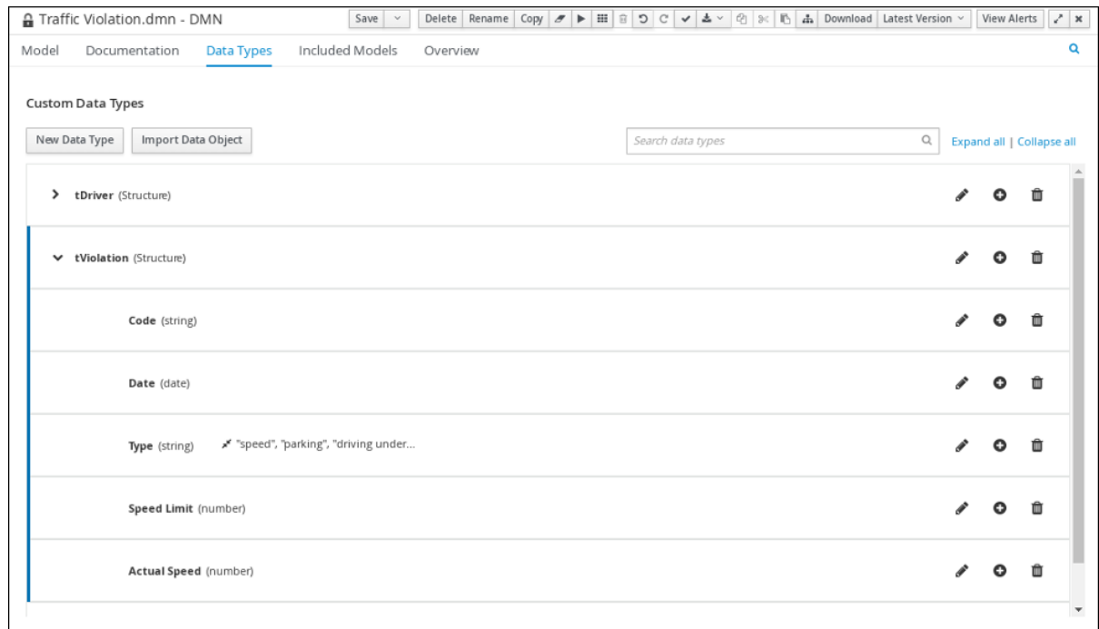
図3.6 tViolation のカスタムデータタイプ
