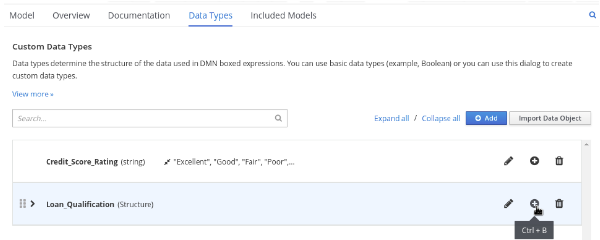
図3.32 新しい構造化データ型へのネスト化フィールドの追加
