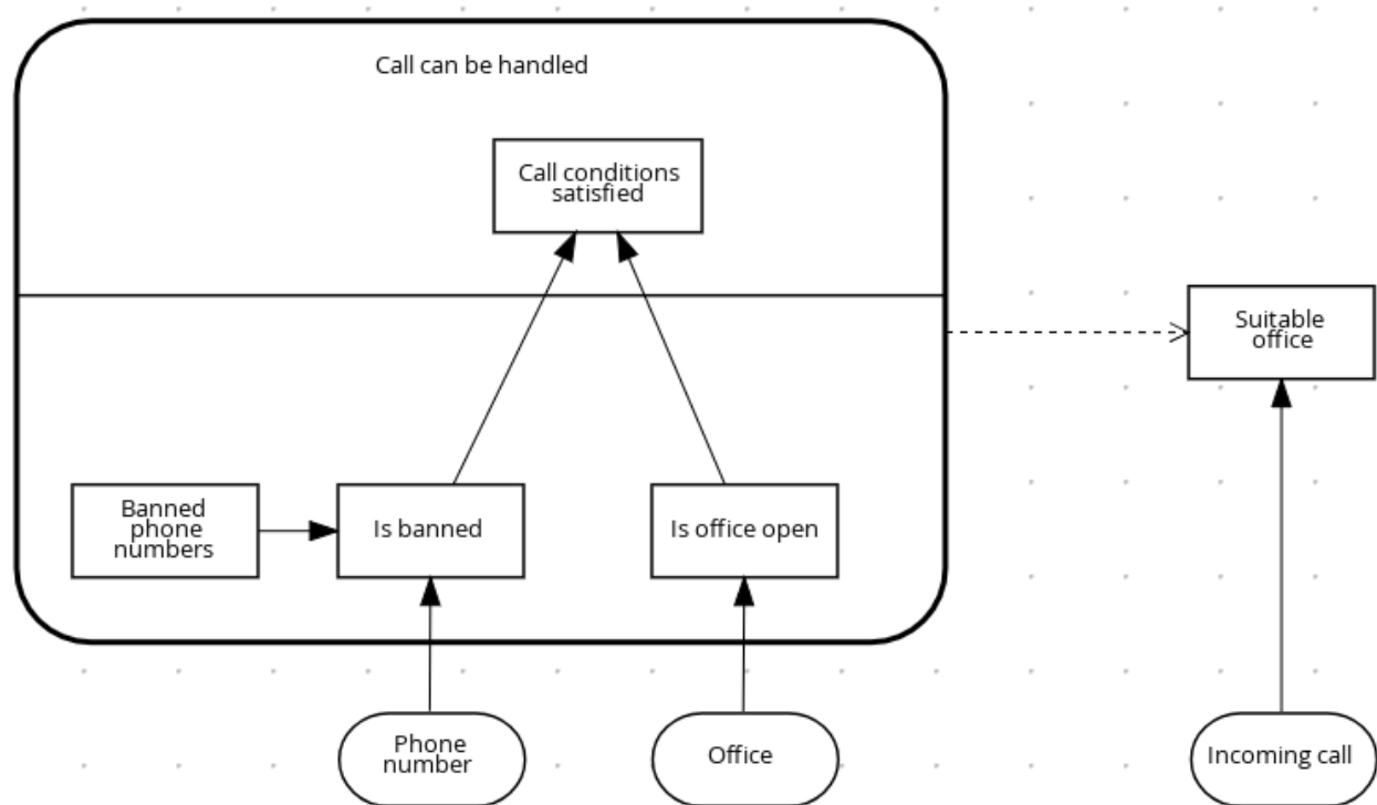
図1.2 DRD 例: デシジョンサービスとしての電話の対応
