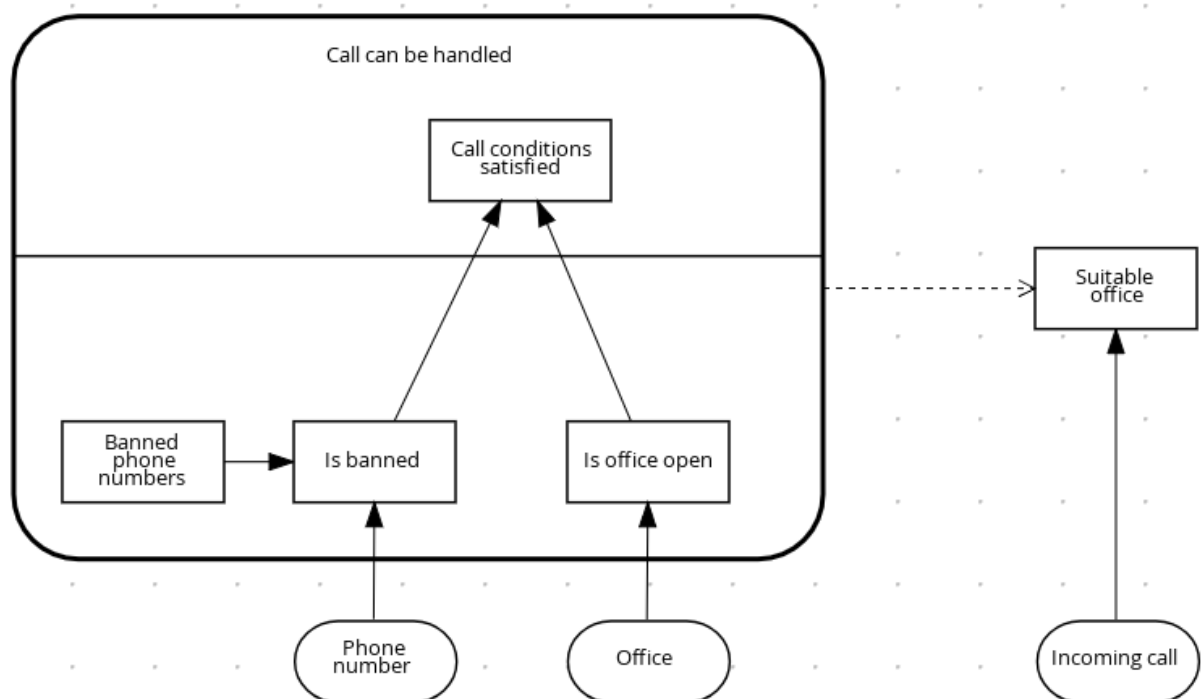
図3.10 デジジョンサービスを使用した電話対応の完全な DRD
