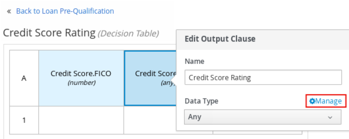
図3.25 列のヘッダー値のデータ型管理
