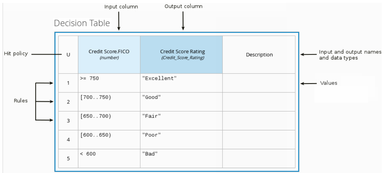
図1.3 クレジットスコア評価のデシジョンテーブル
