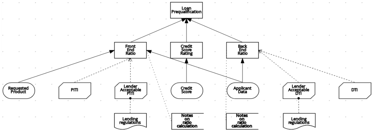
図1.1 DRD 例: ローンの前審査
