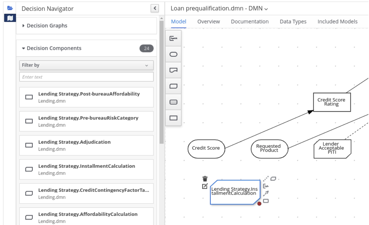
図3.42 追加した DMN モデルの DRD コンポーネントの追加
