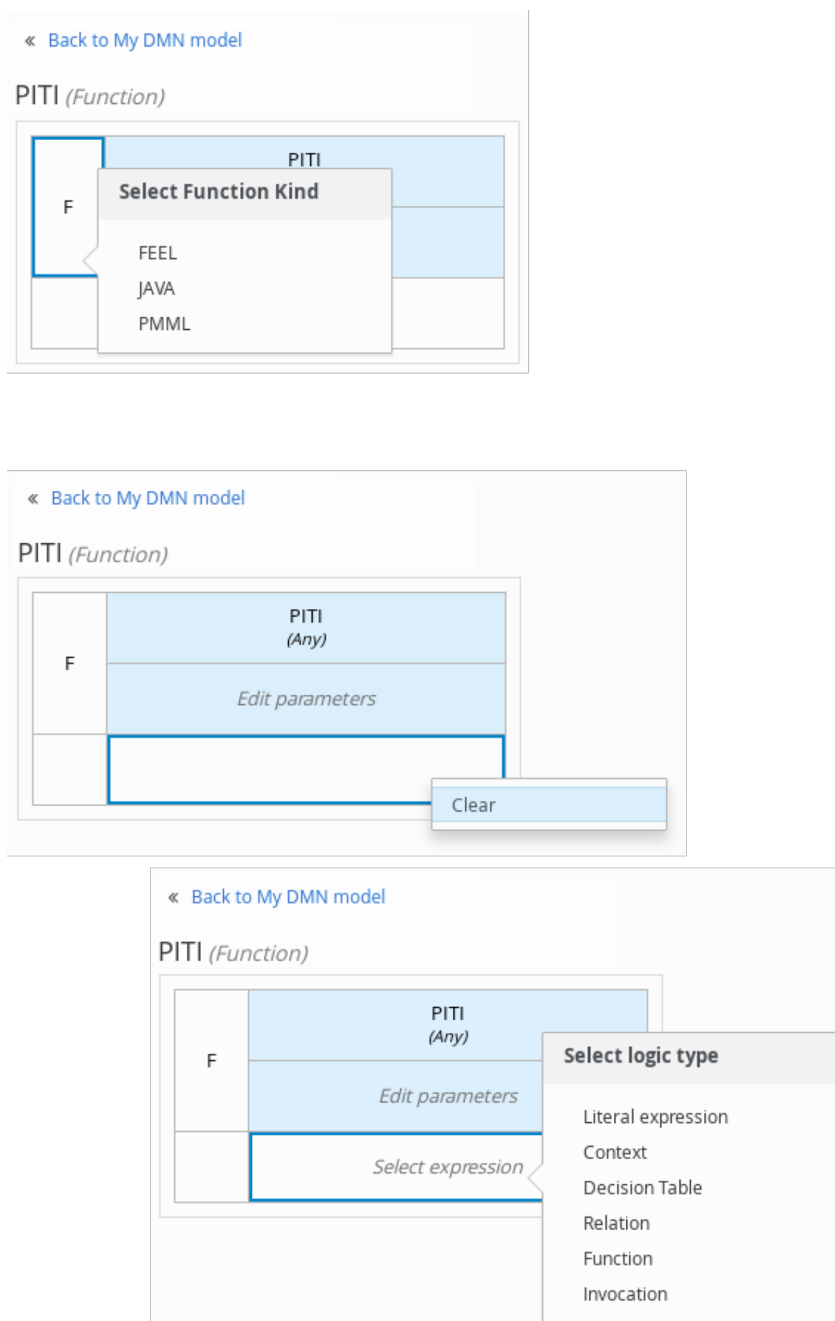
図3.5 ビジネスナレッジモデルの機能または他のロジックタイプの選択
