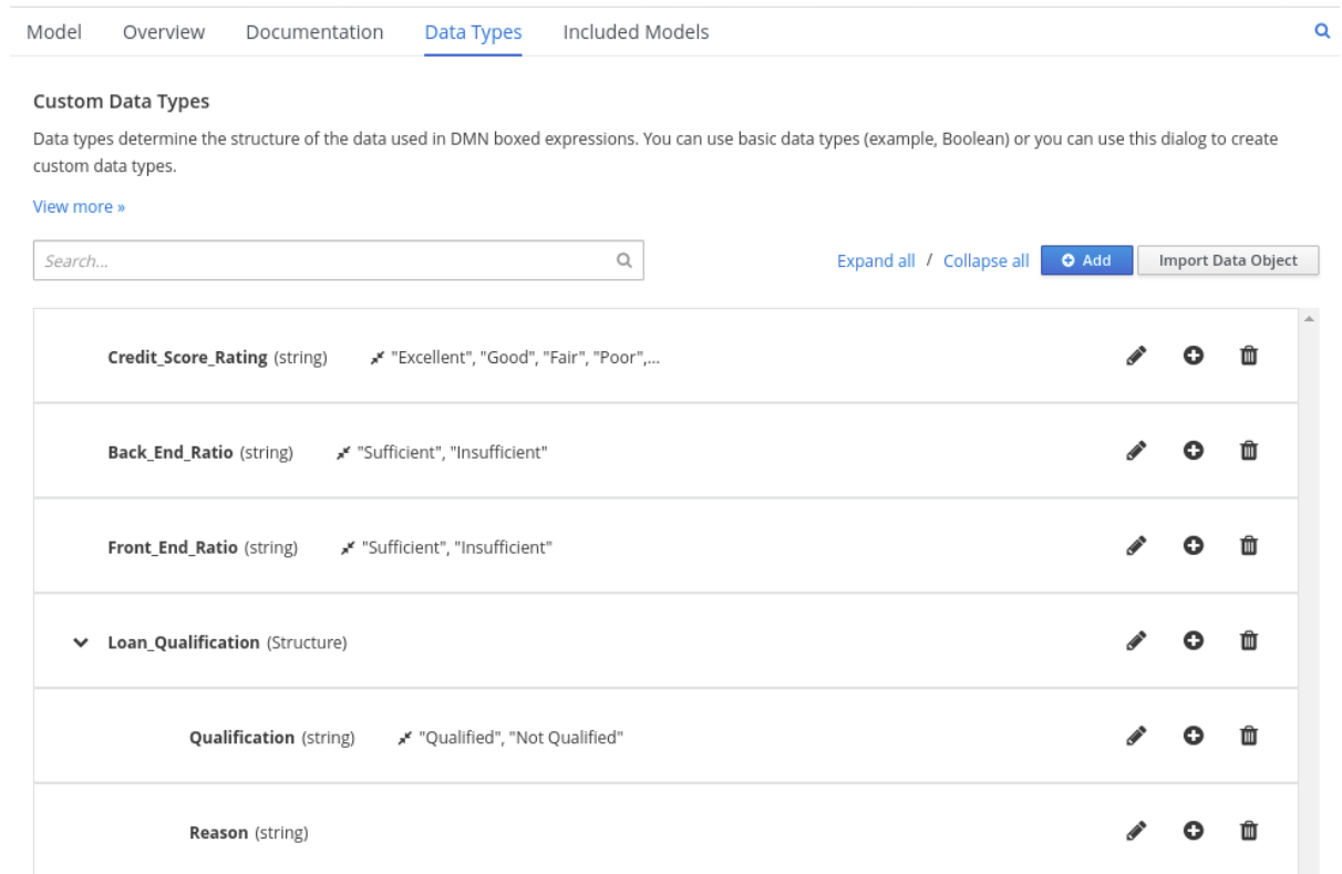
図3.33 ネスト化されたデータ型への制約の追加
