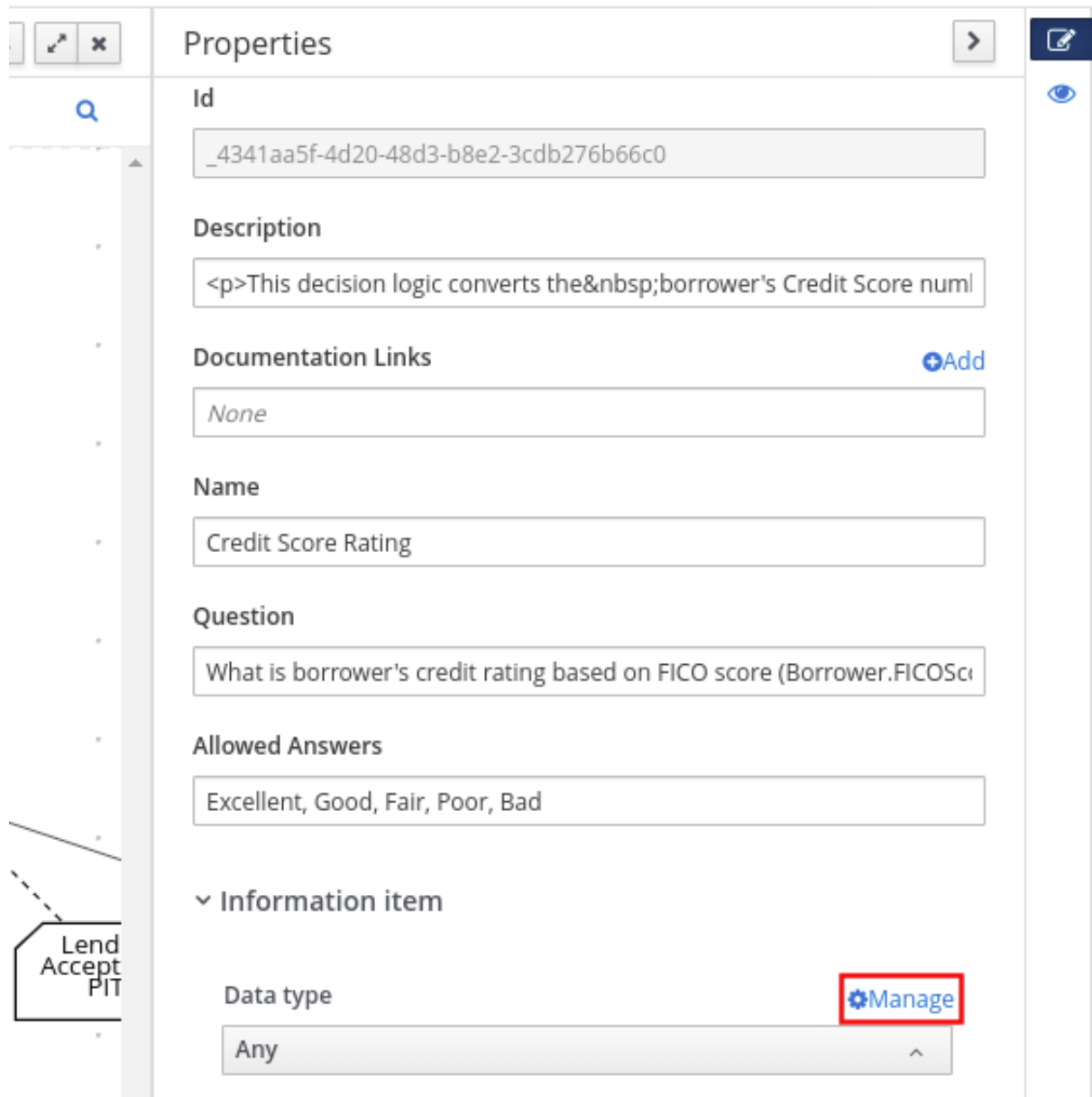
図3.26 意思決定要件 (DRD) プロパティでのデータ型の管理
