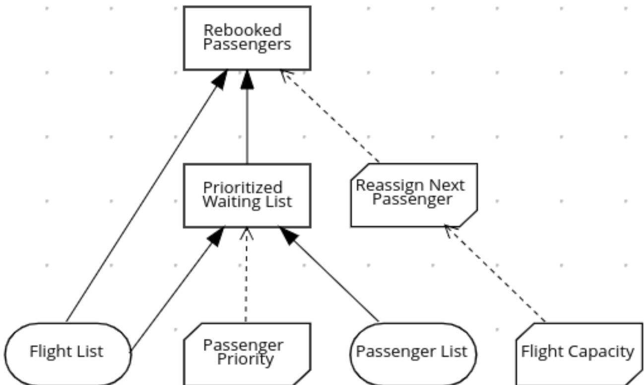
図1.17 フライト予約変更の DRD
