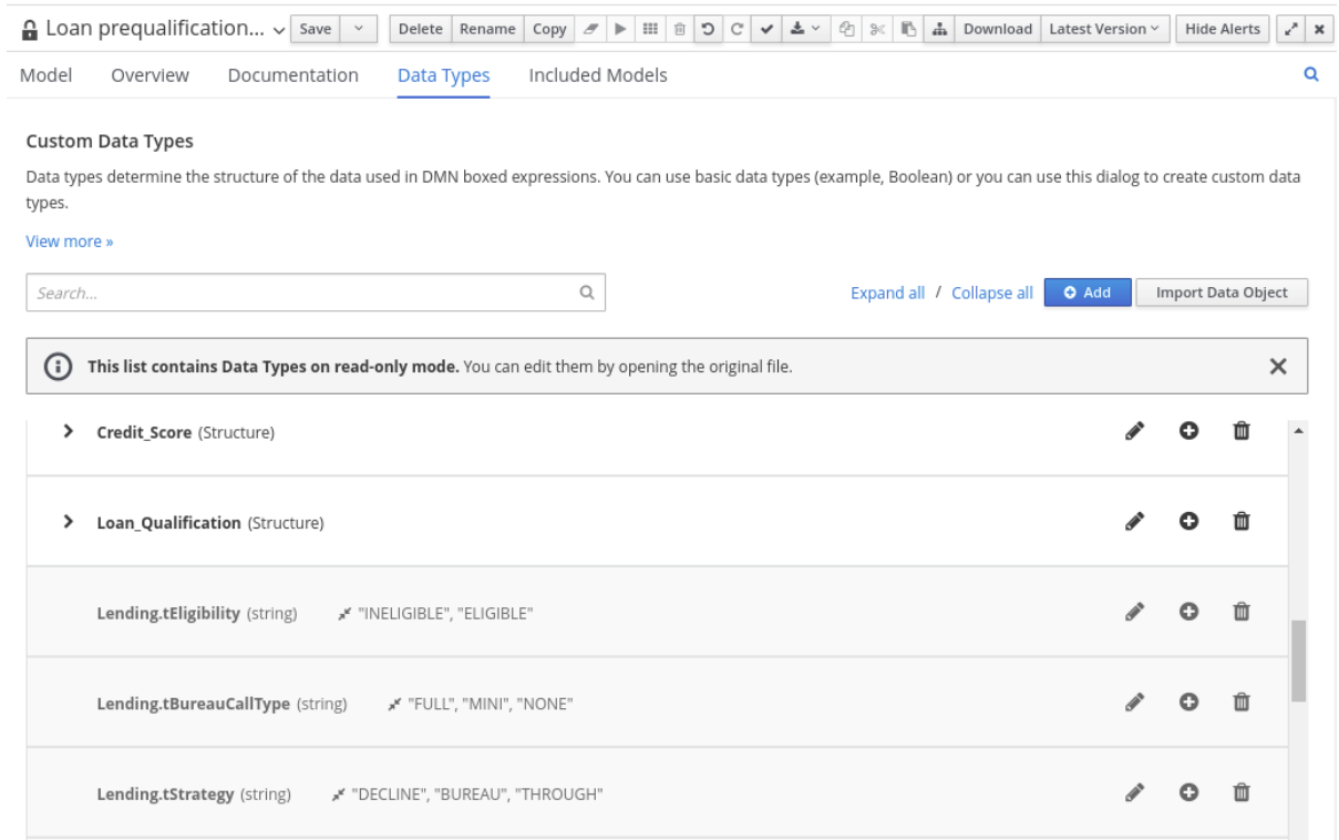
図3.41 追加した DMN モデルのデータ型を含む DMN ファイル
