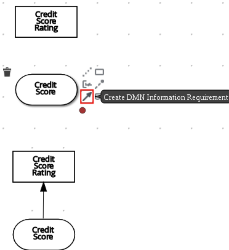
図3.8 クレジットスコアの入力からクレジットスコア評価のデシジョンへの接続
