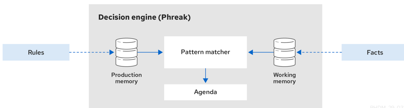
図1.1 基本となるデシジョンエンジンコンポーネントの概要
