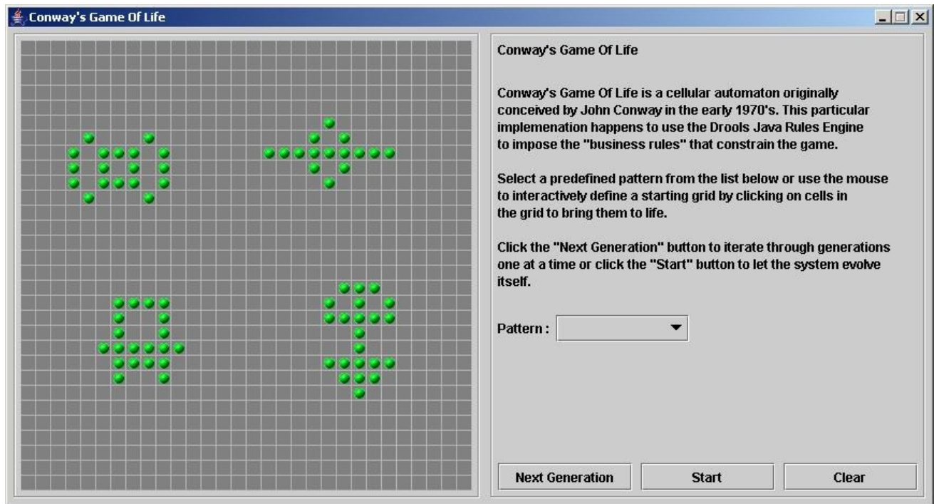
図9.25 Conway の例の世代進化
