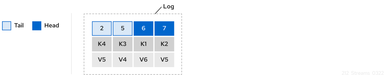
図3.2 コンパクション後のログ
