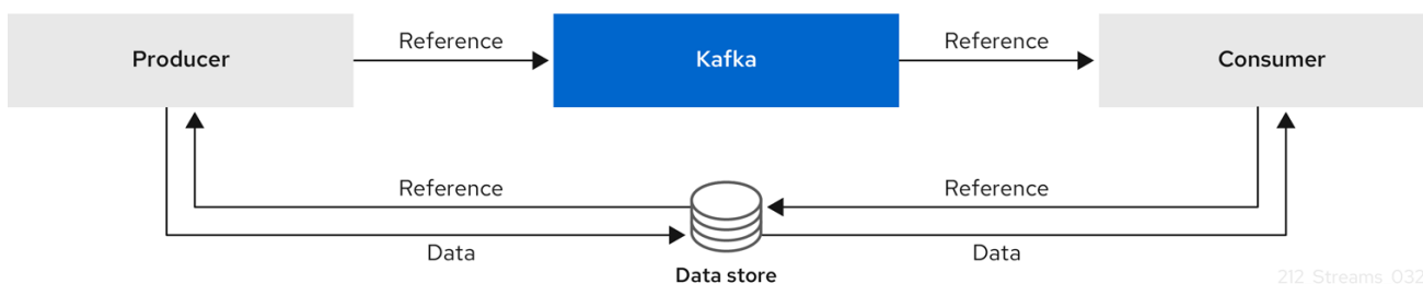
図3.4 参照ベースのメッセージングフロー
