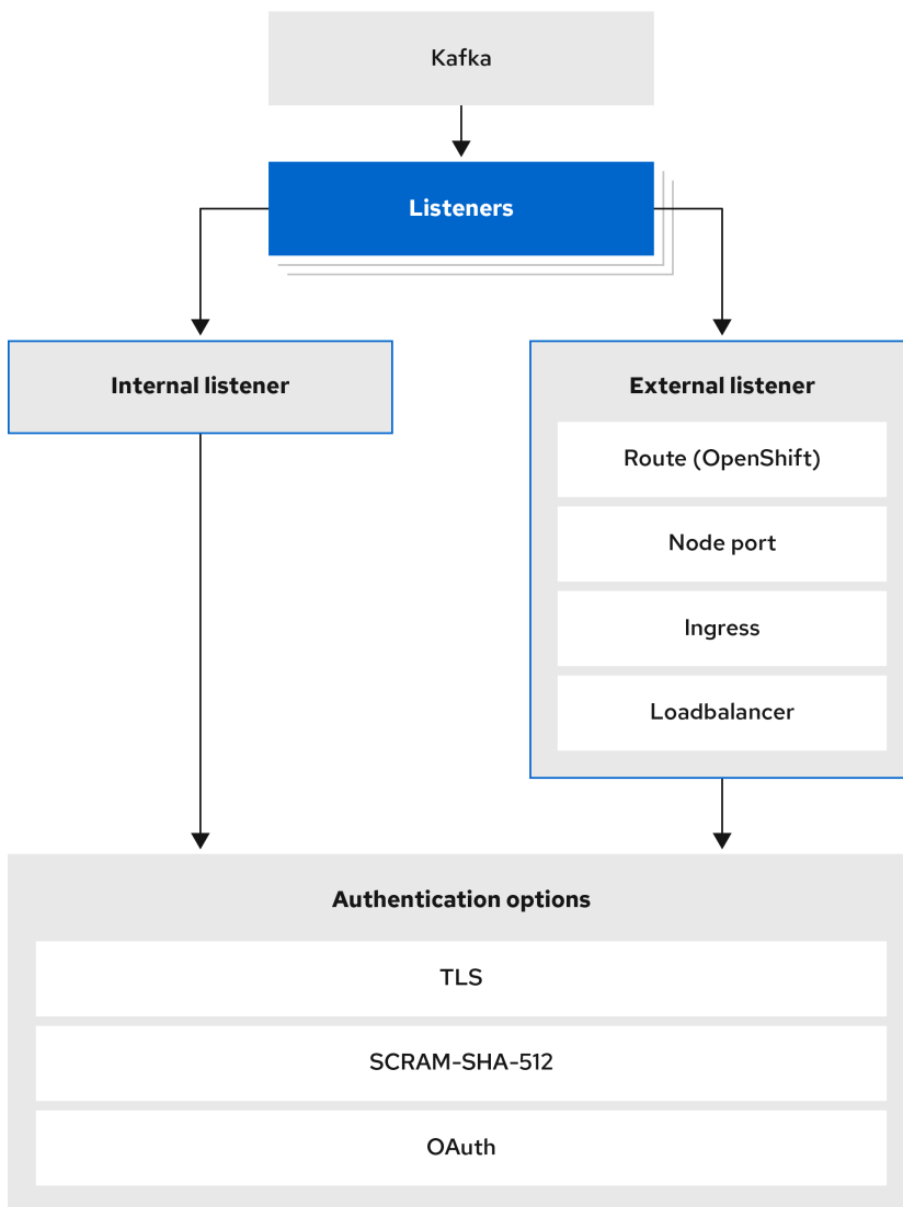
図4.1 Kafka リスナーの認証オプション
