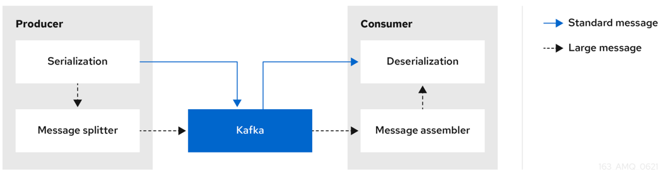
図12.5 インラインメッセージングフロー
