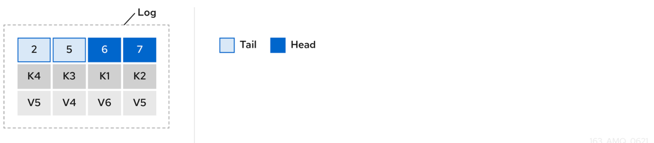
図12.2 コンパクション後のログ
