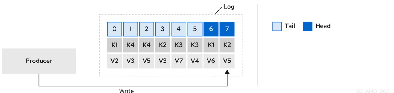
図12.1 コンパクション前のオフセットの位置によるキー値の書き込みを示すログ
