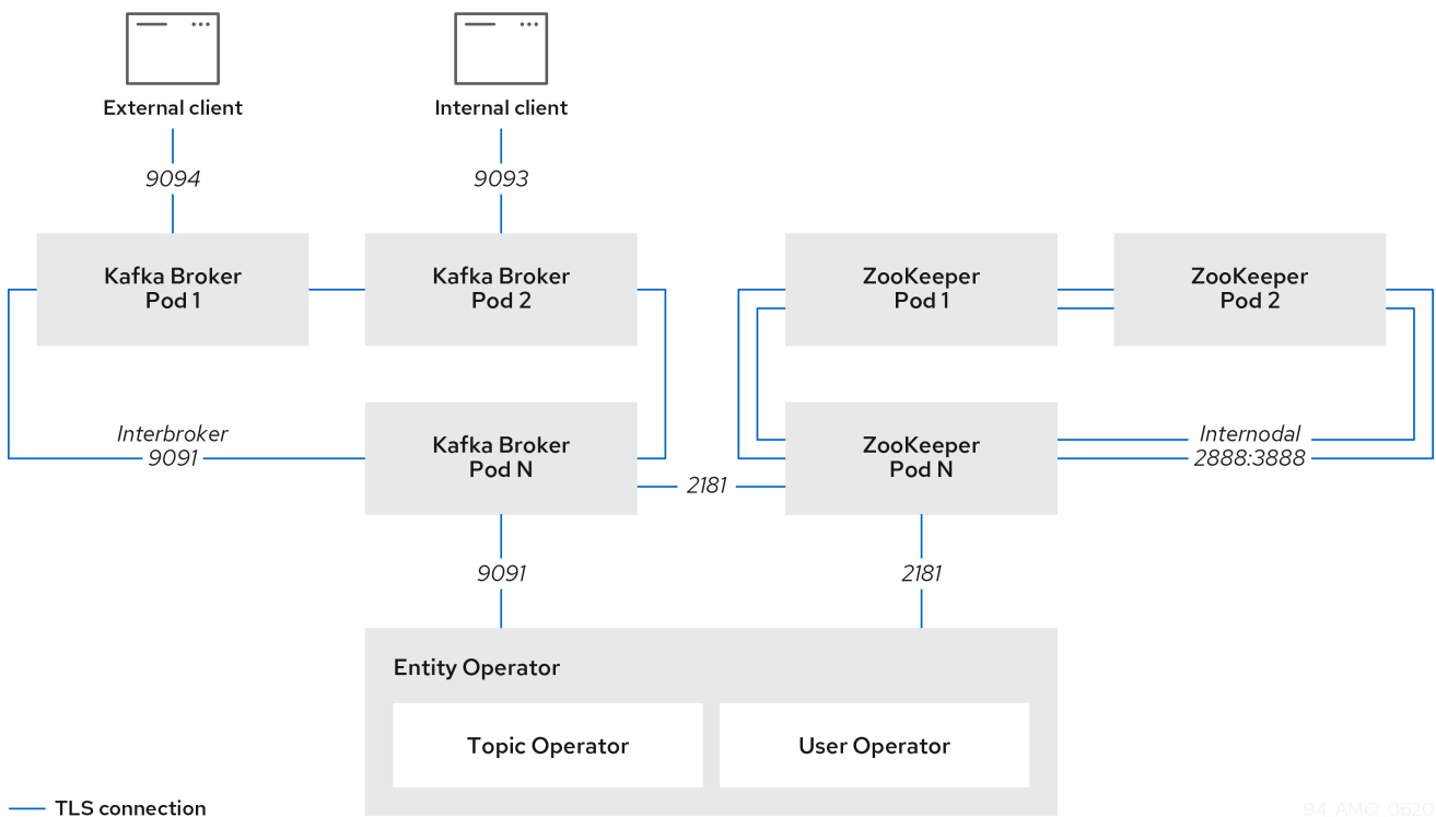
図11.1 TLS によってセキュリティーが保護された通信のアーキテクチャー例
