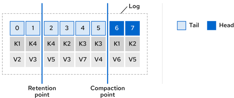
図12.3 ログ保持ポイントおよびコンパクションポイント
