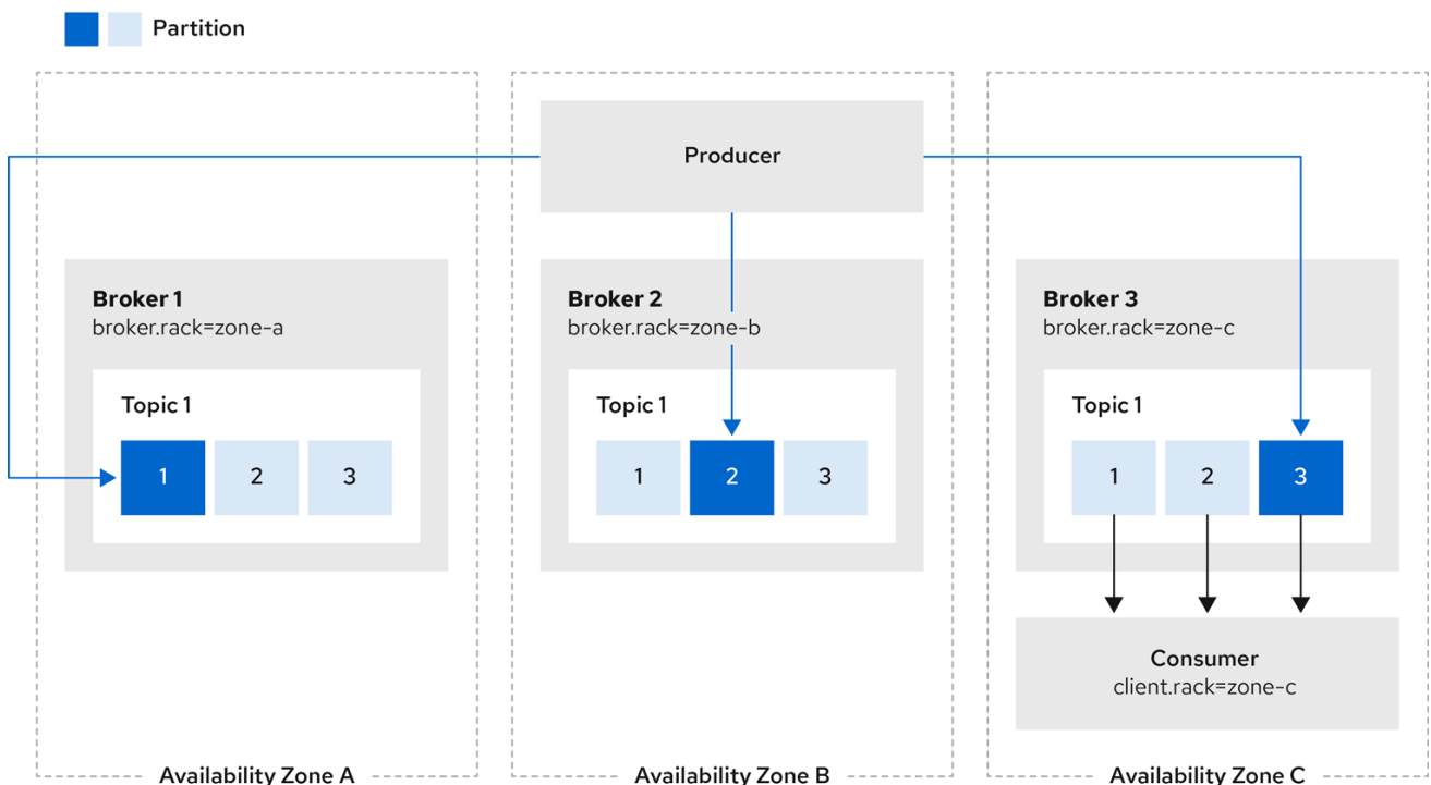
図13.1 同じアベイラビリティゾーンのレプリカから消費するクライアントの例
