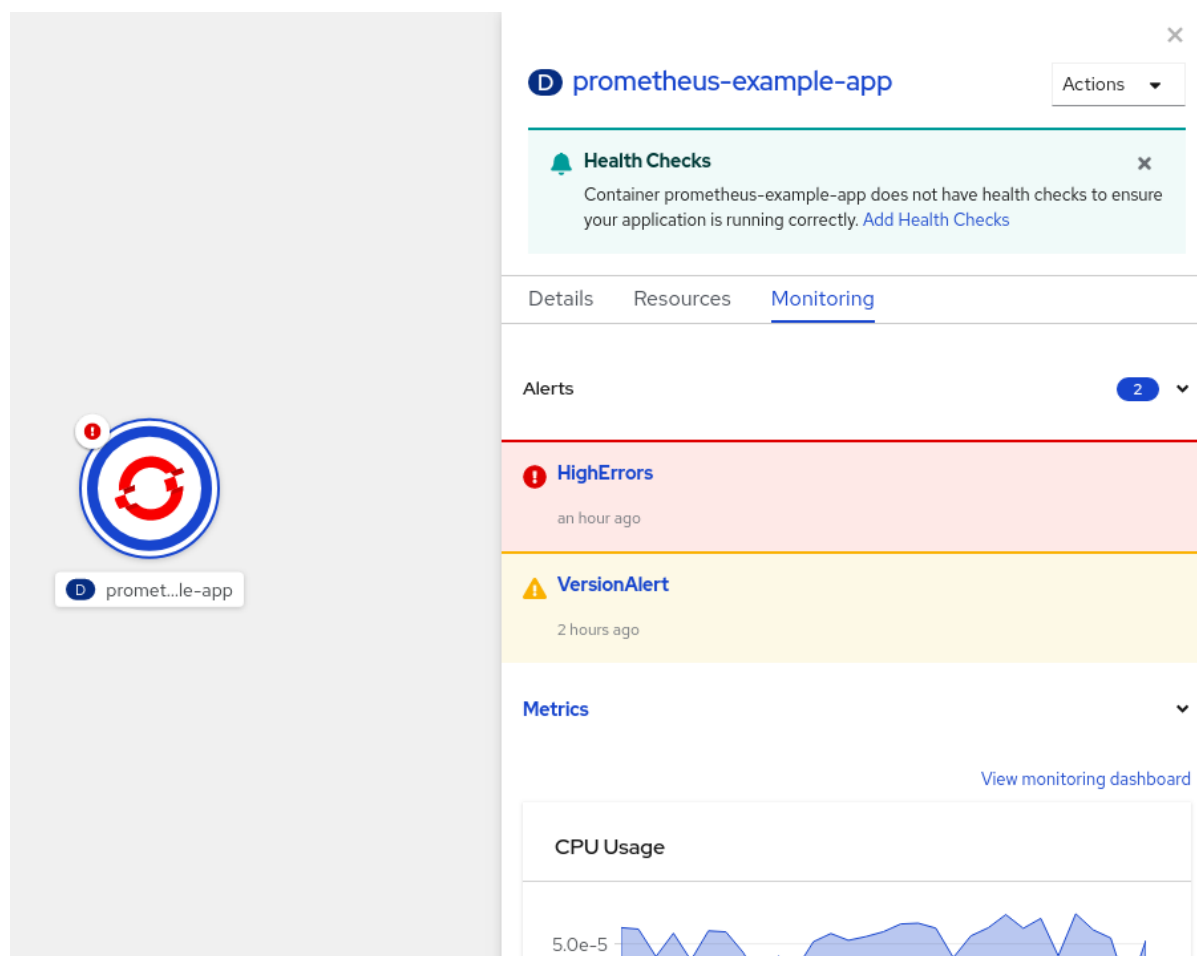
図10.5 アプリケーションメトリクスのモニタリング
