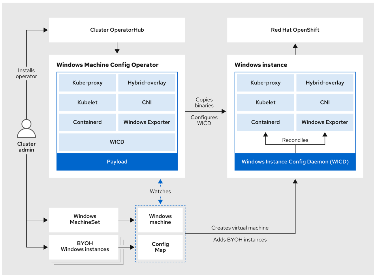
図3.1 WMCO の設計
