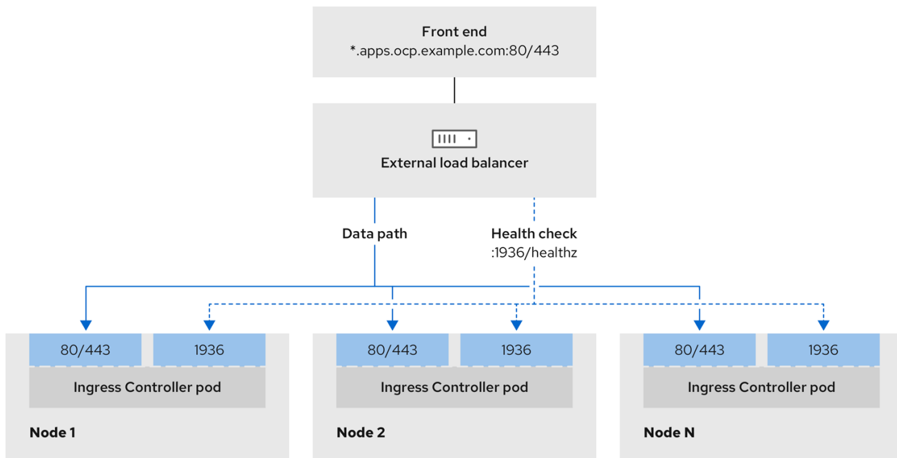
図23.4 OpenShift Container Platform 環境で動作する Ingress Controller を示すネットワークワークフローの例
