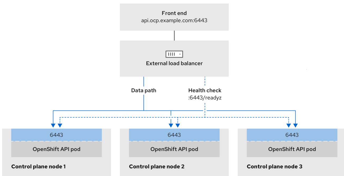
図23.5 OpenShift Container Platform 環境で動作する OpenShift API を示すネットワークワークフローの例
