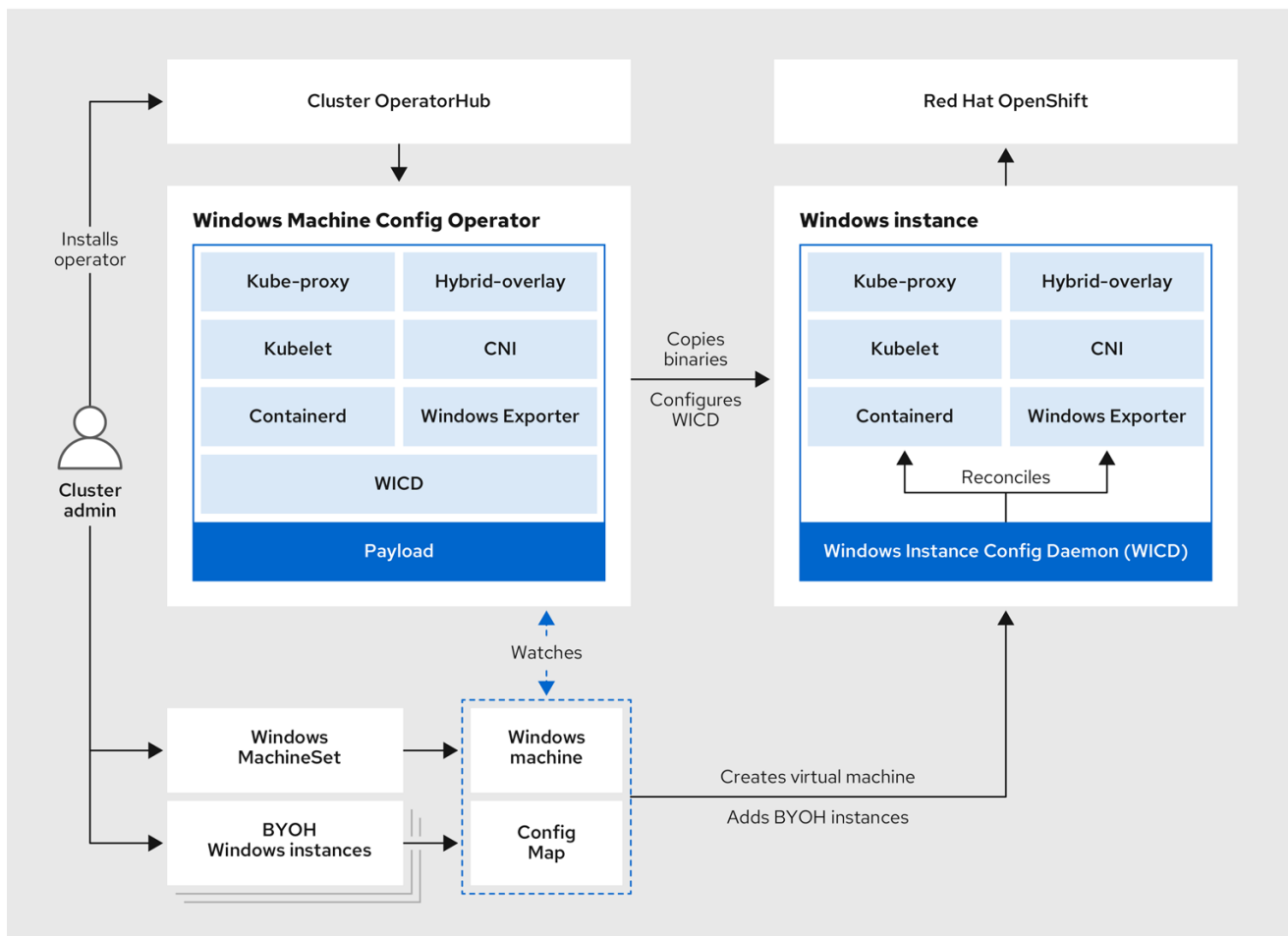
図3.1 WMCO の設計
