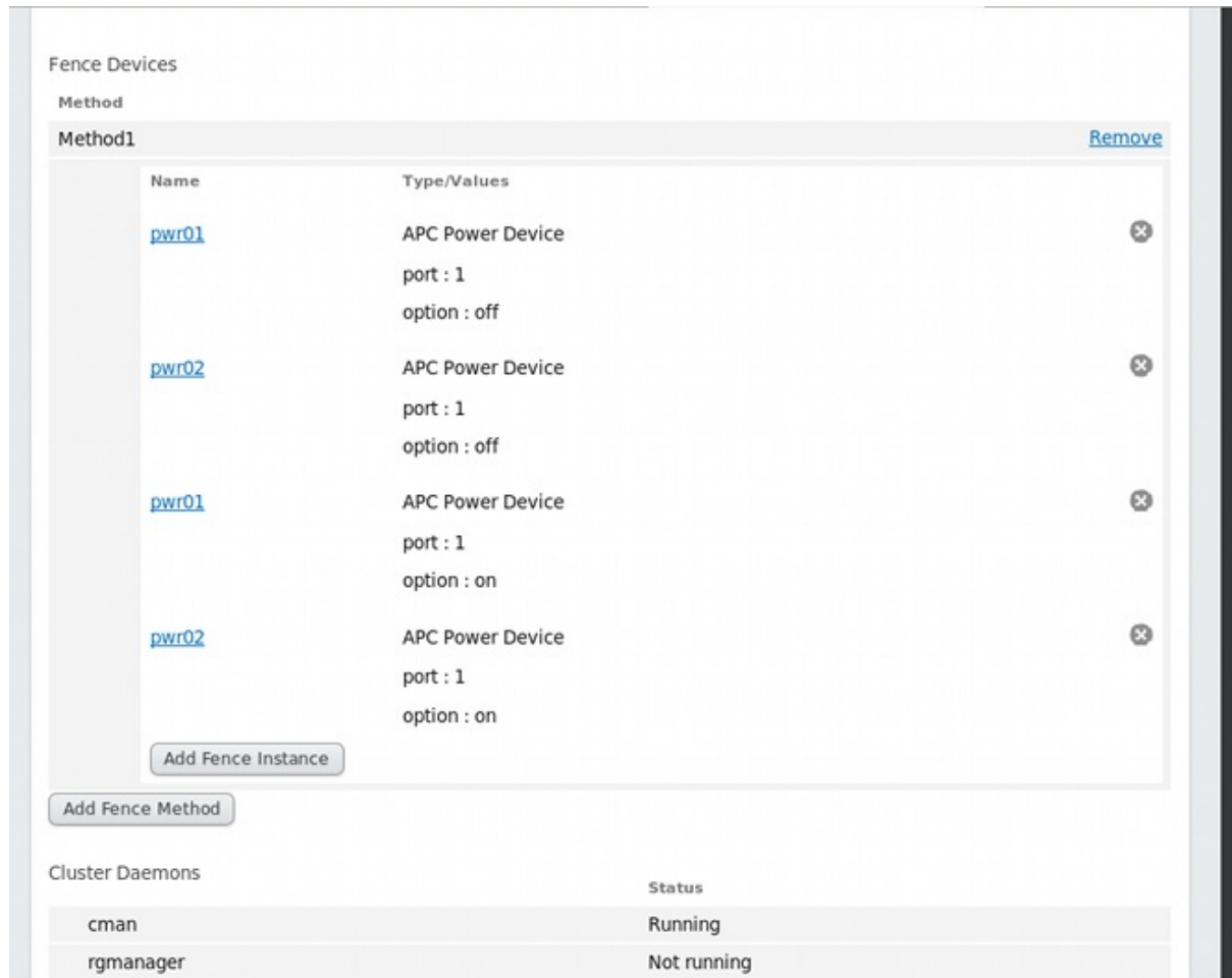
Figura 3.6. Configuración de cercado de doble energía
